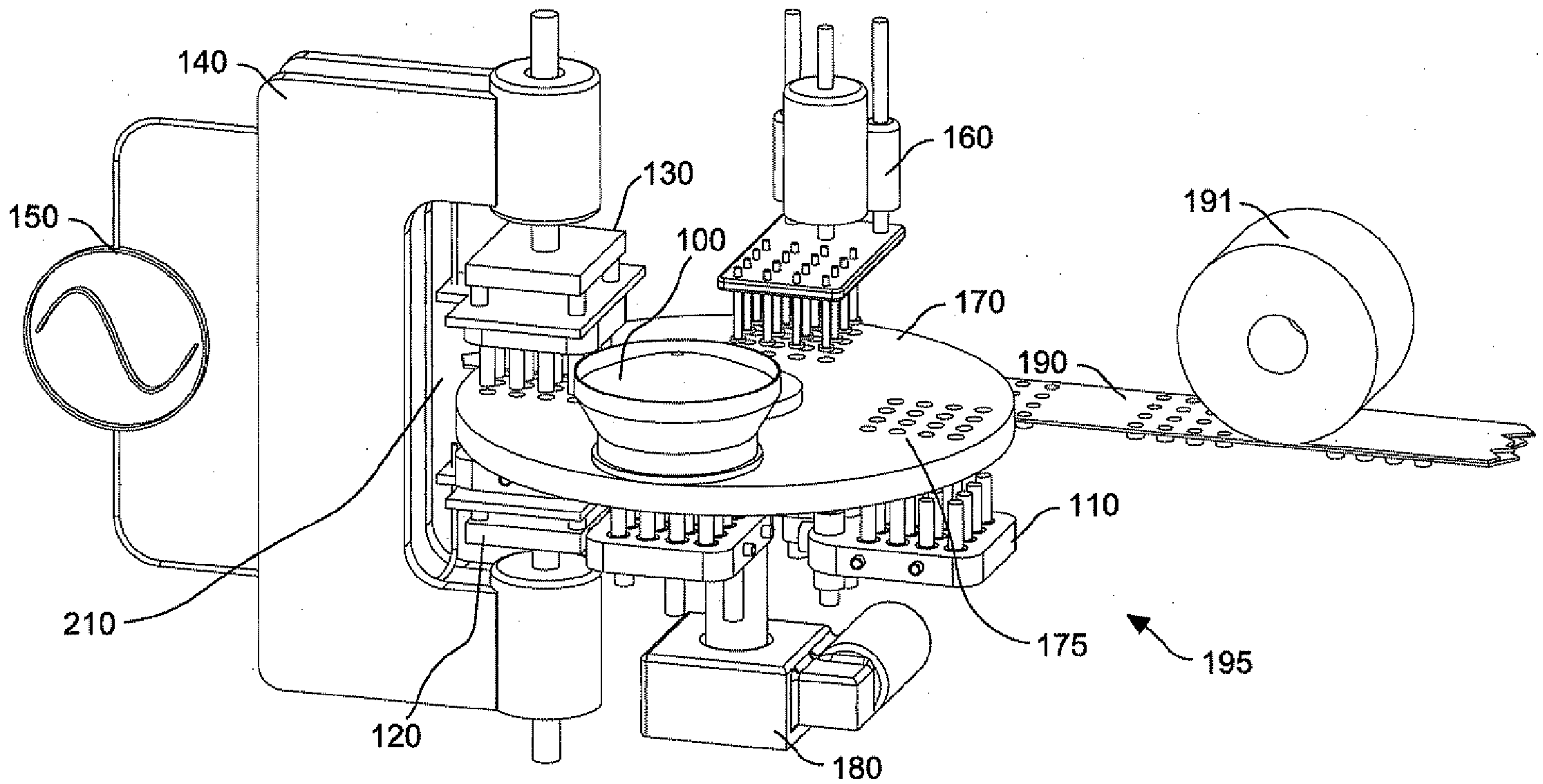
FIG. 4A
