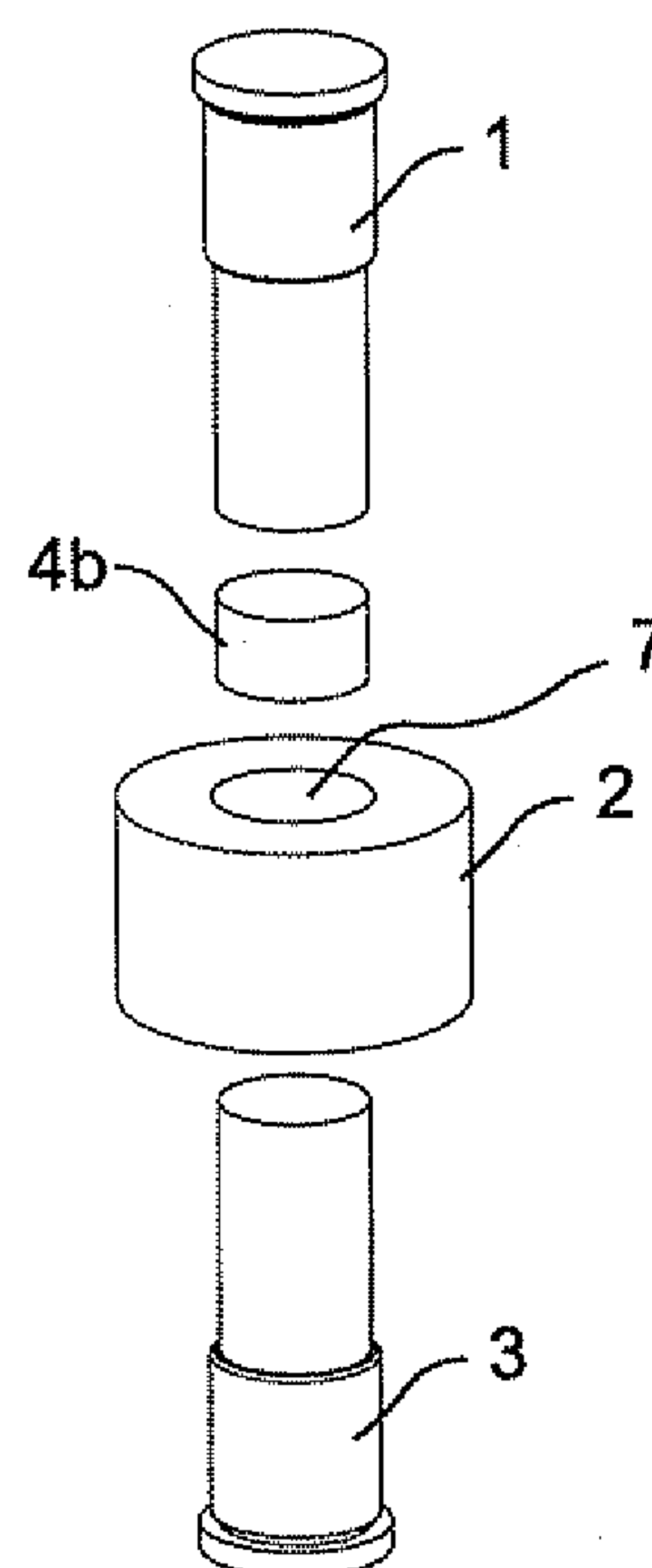
FIG. 1F
