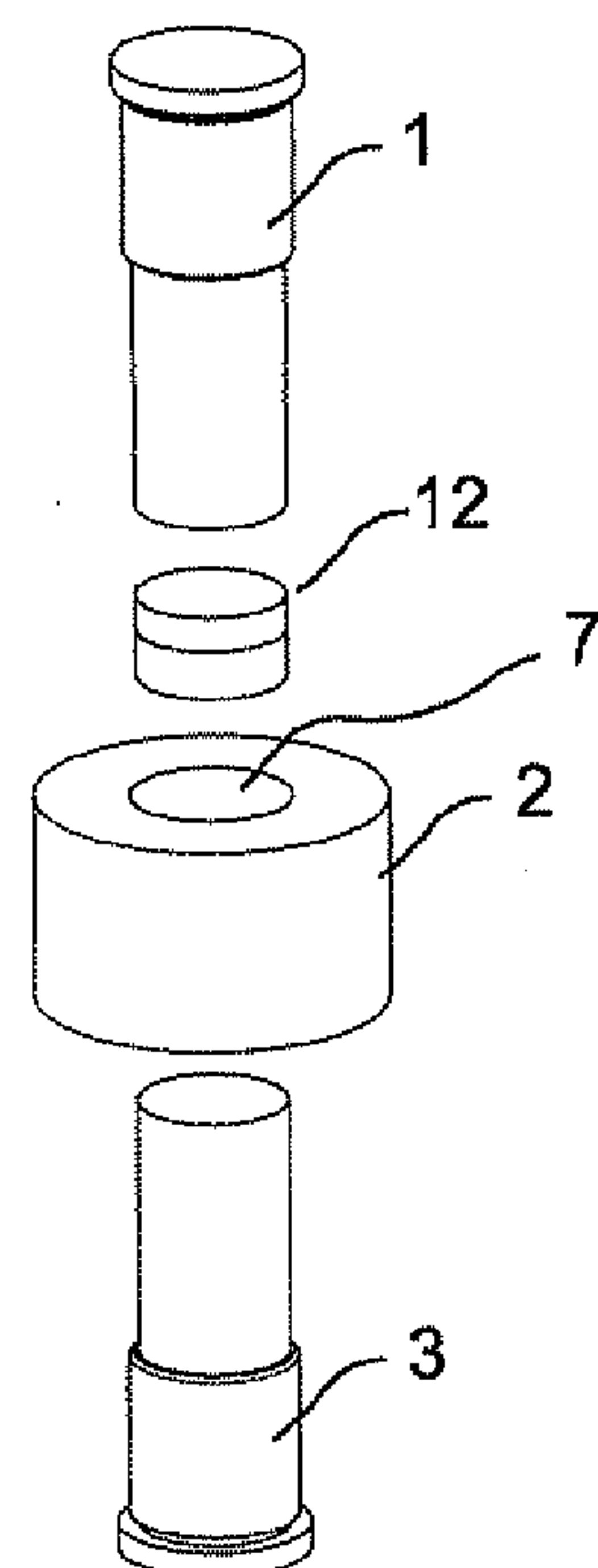
FIG. 2H
