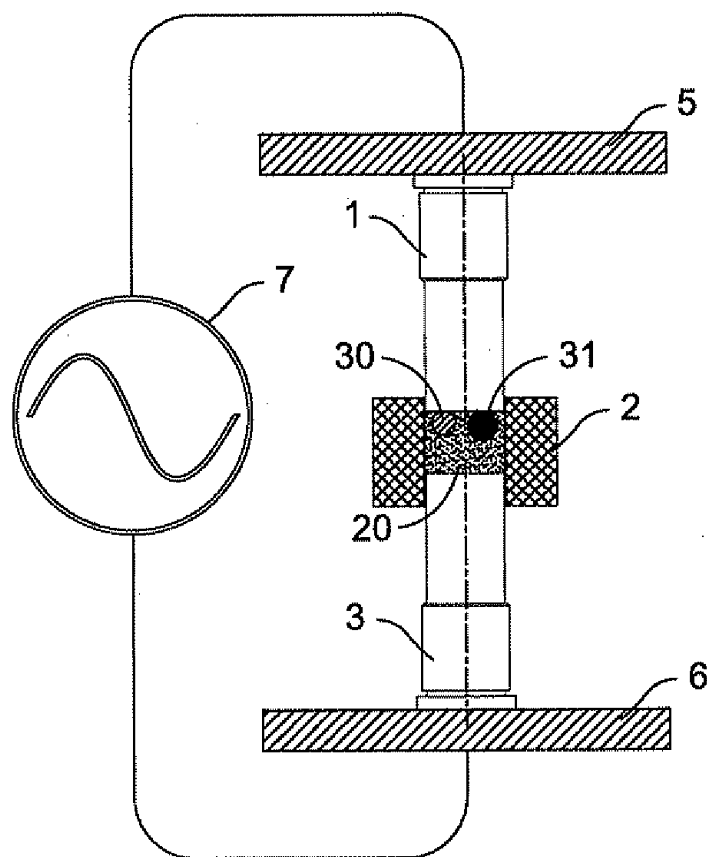
FIG. 3E
