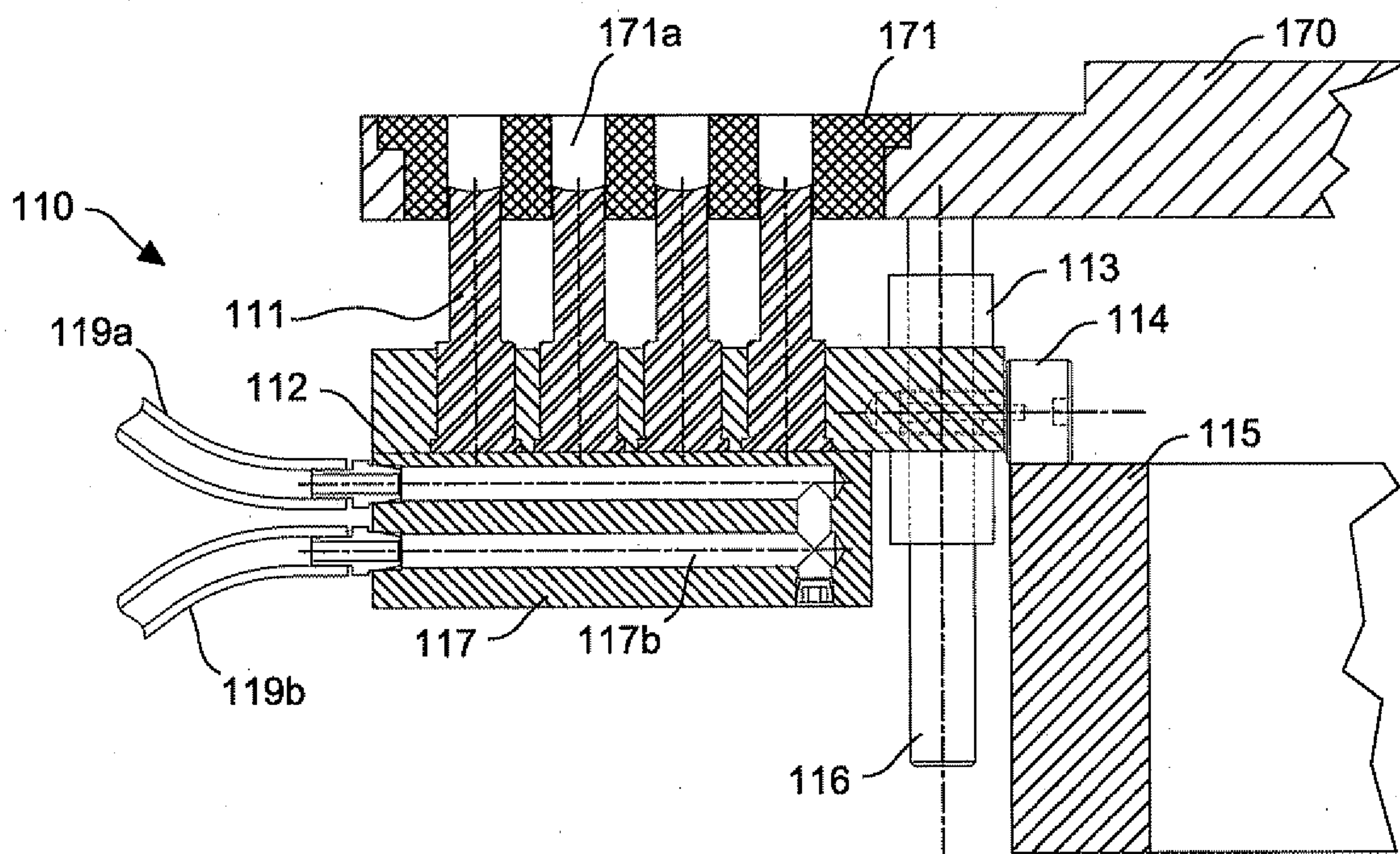
FIG. 6A
