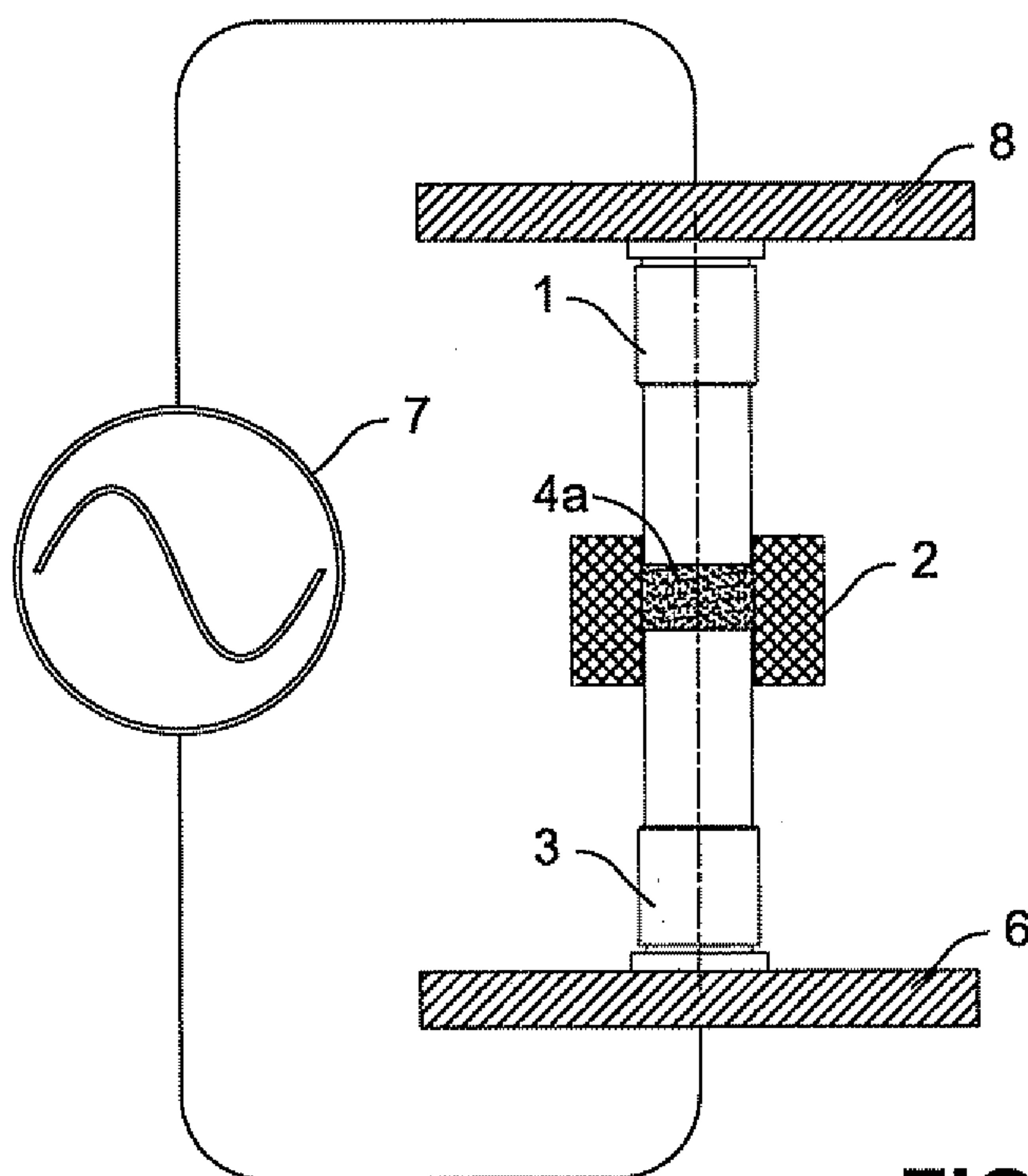
FIG. 1C
