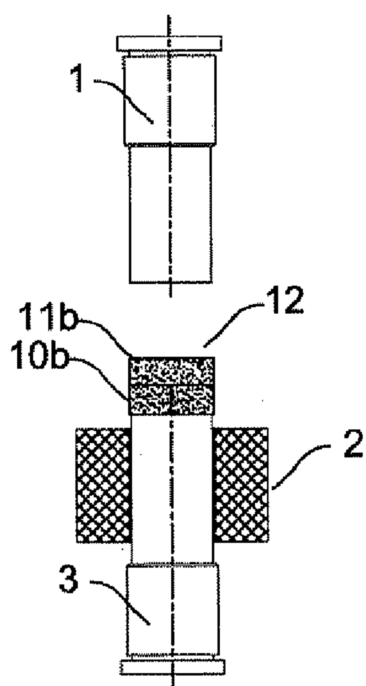
FIG. 2G
