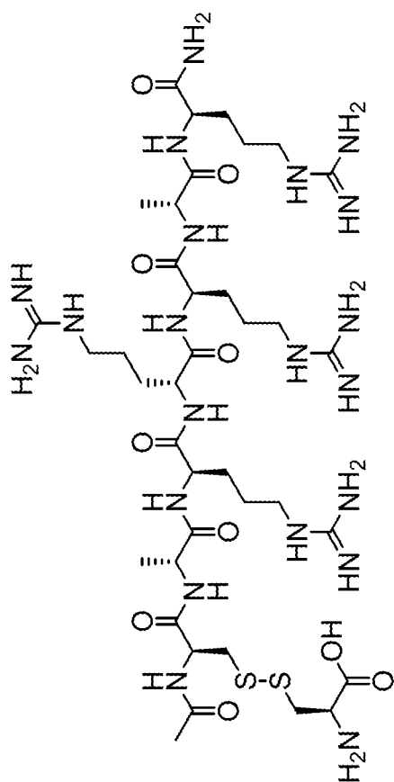
Ac-D-Cys(L-Cys-OH)-D-Ala-D-Arg-D-Arg-D-Arg-D-Arg-D-Ala-D-Arg-NH 2
