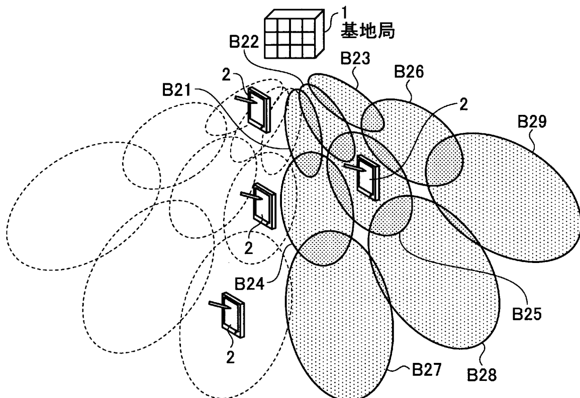
(b)2回目のビーム照射方向(照射パターンB2)
