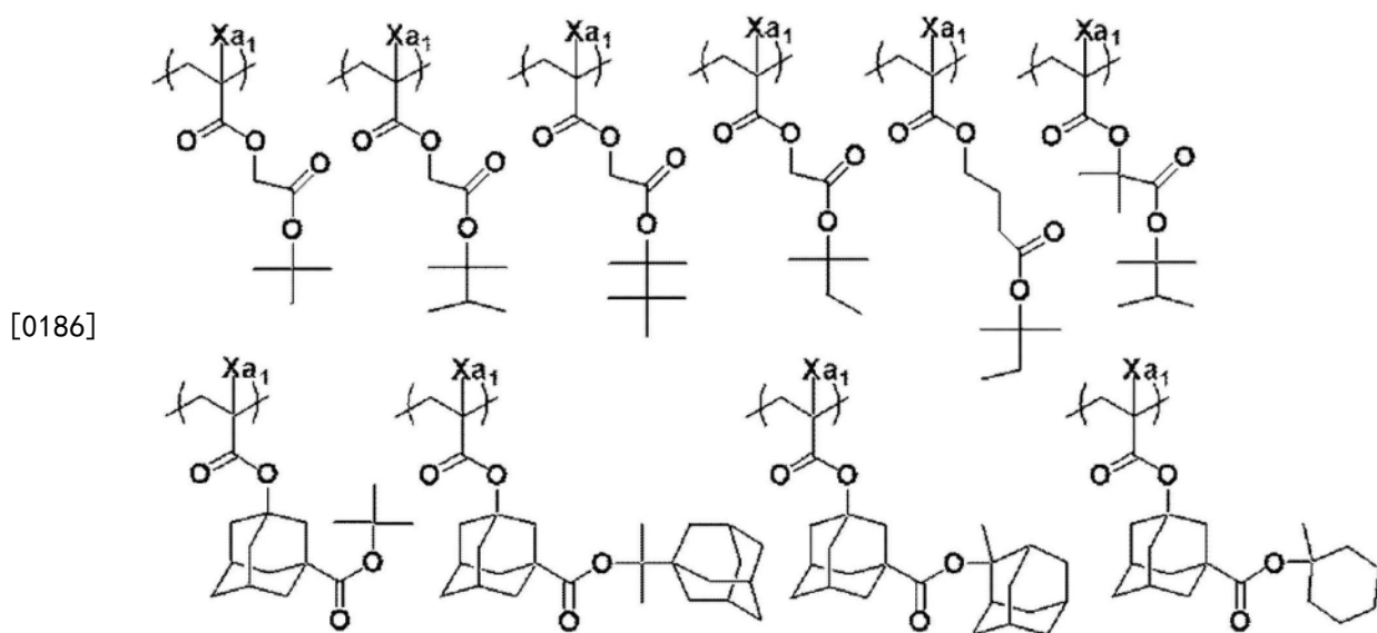
[0187] [化学式7]
