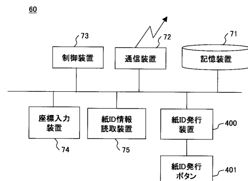
筆記情報入力装置を示す図
