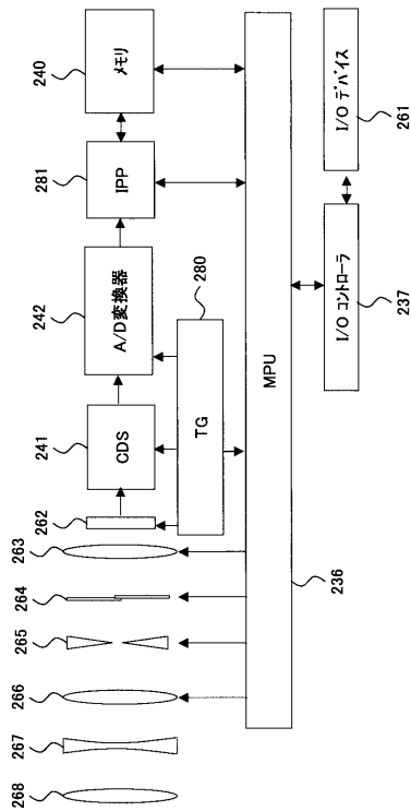
撮像部の構成例を示す図
