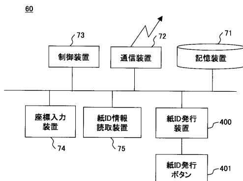
筆記情報入力装置を示す図
