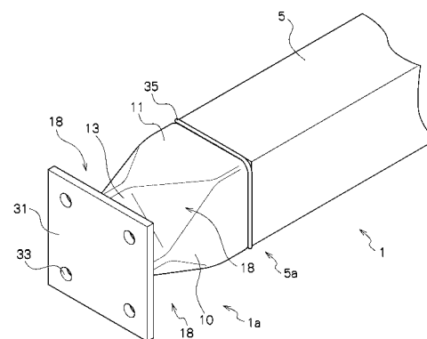
1: 角形鋼管部材 5: 角形鋼管 11: 溶接接合部 18: 締結作業用空間 33: ボルト孔 4: 鋼製中空ジョイント 10: ジョイント本体 13: プレート接合部 31: エンドプレート
