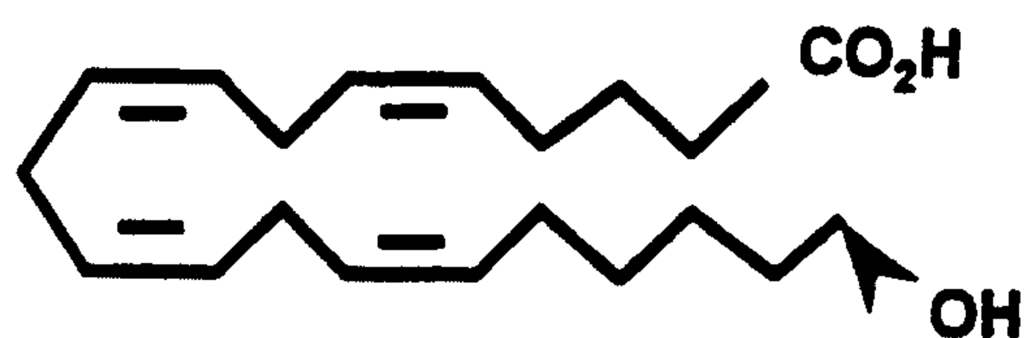
20-HETE
