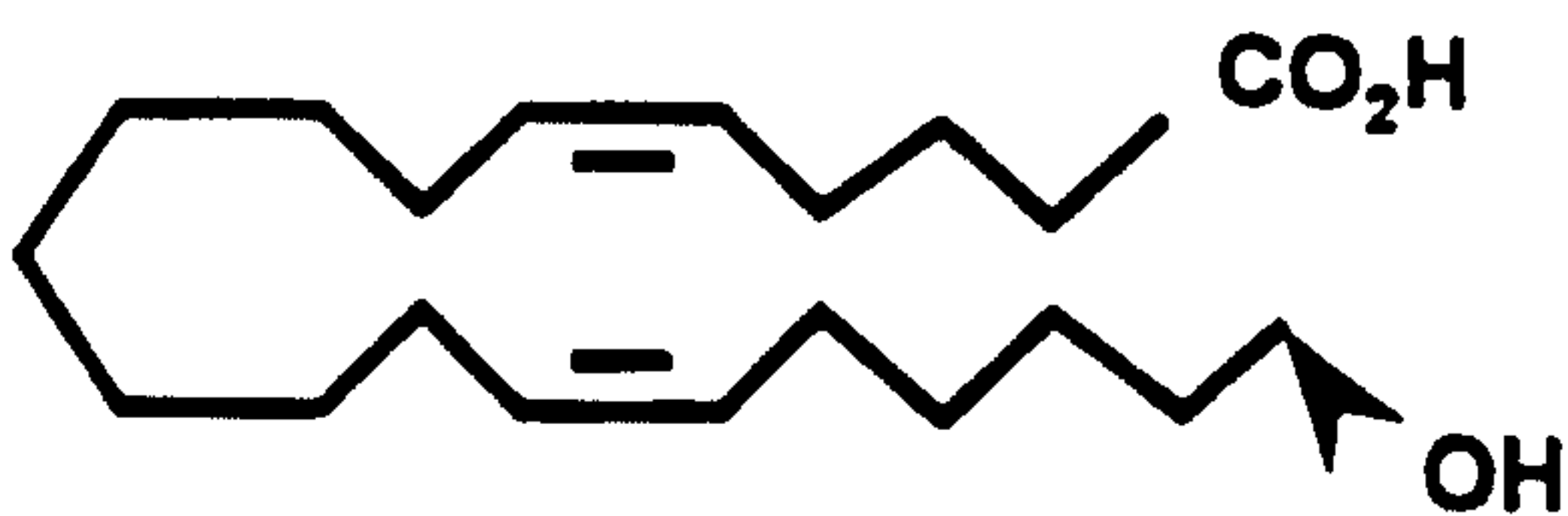
ps 20-HETE
