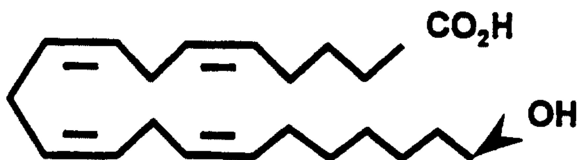
21-HETE
