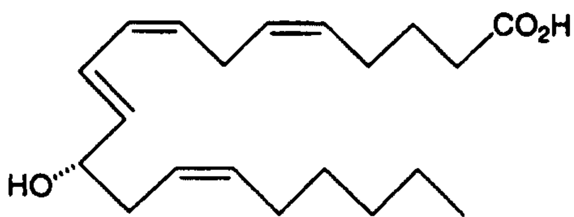
12(S)-HETE
