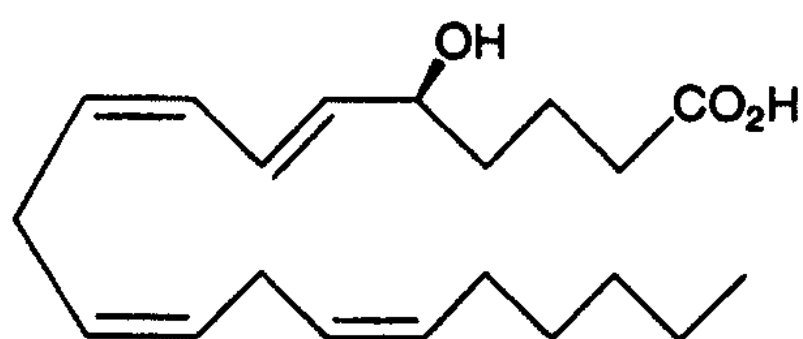
5(S)-HETE
