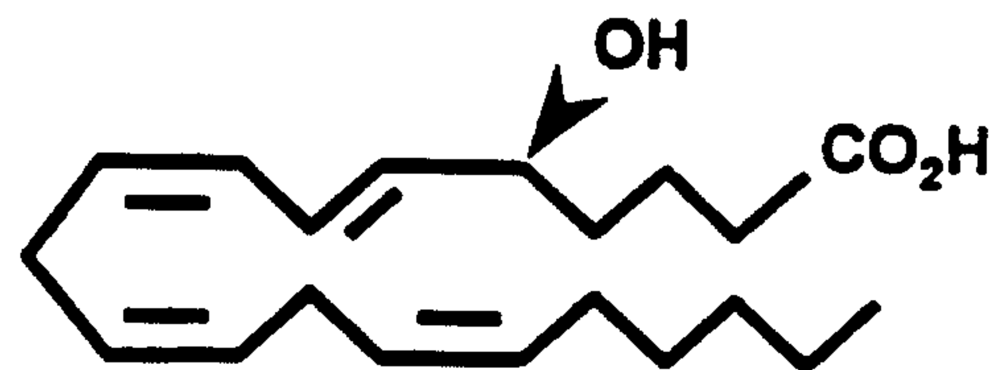
5(S)-HETE
