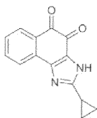
Composé 13
