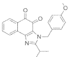
Composé 30
