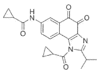
Verbindung 21
