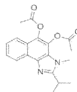
Composé 184
