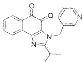
Verbindung 82
