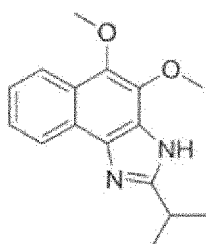
Verbindung 188
