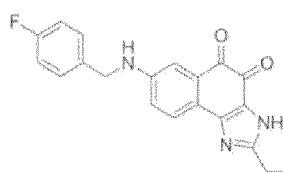
Composé 46
