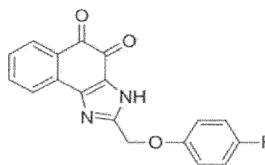
Verbindung 78
