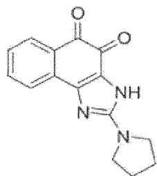
Verbindung 62
