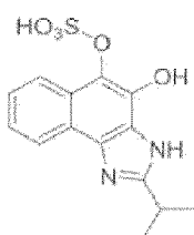
Composé 179
