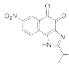
Composé 15
