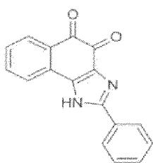
Composé 4
