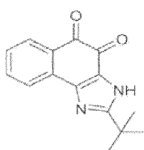
Composé 5
