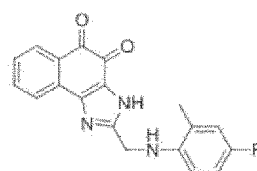
Verbindung 52
