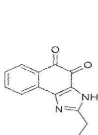
Verbindung 10
