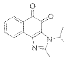
Composé 89
