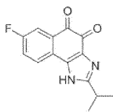
Verbindung 97
