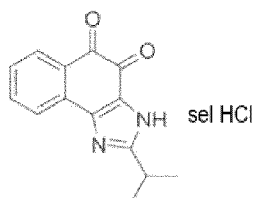
Composé 93
