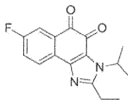
Verbindung 88
