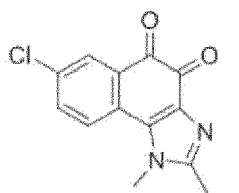
Verbindung 42
