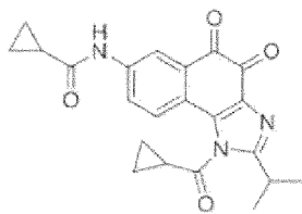
Composé 21
