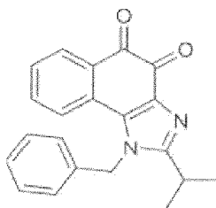
Composé 2
