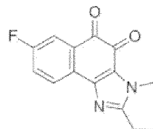
Composé 40
