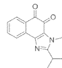
Composé 35
