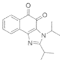
Composé 84
