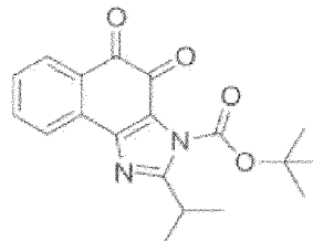
Composé 28
