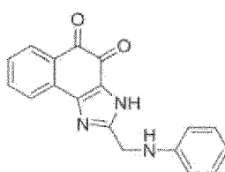
Verbindung 48
