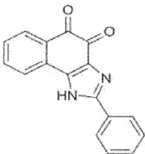
Verbindung 4
