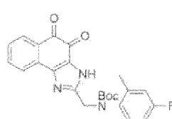
Composé 51
