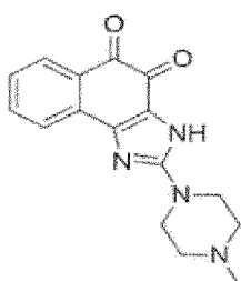
Verbindung 74
