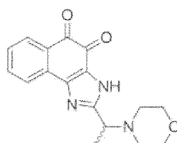
Composé 60
