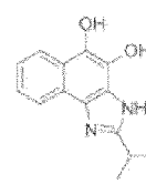
Composé 175
