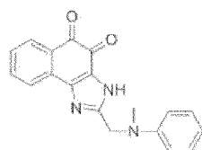
Composé 50
