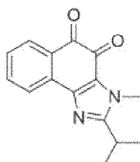
Verbindung 34
