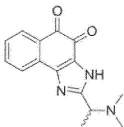
Verbindung 59
