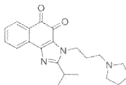
Composé 57
