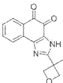
Verbindung 98
