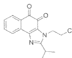
Composé 63
