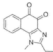
Verbindung 38
