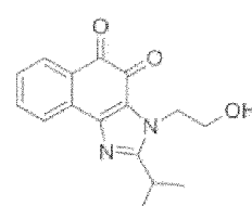
Composé 67
