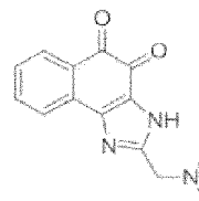
Composé 58
