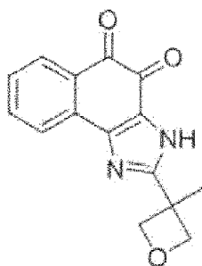
Verbindung 98
