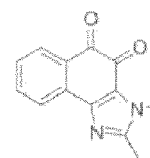
Composé 95
