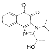
Verbindung 90
