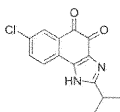
Verbindung 16
