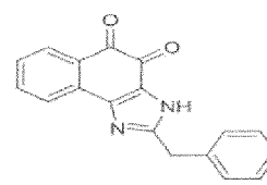
Composé 12
