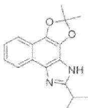
Composé 185
