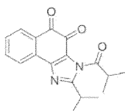
Composé 24
