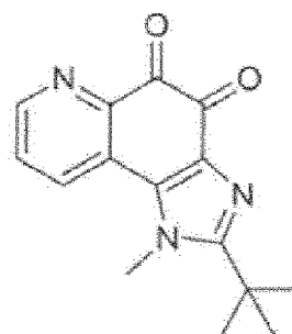
Verbindung 9
