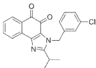
Verbindung 33
