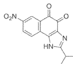
Verbindung 15
