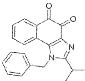
Verbindung 2
