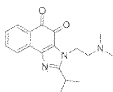
Composé 71
