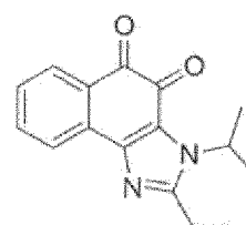
Verbindung 89
