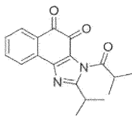
Verbindung 28
