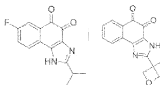
Composé 97
