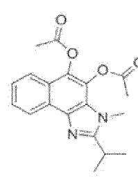
Verbindung 184
