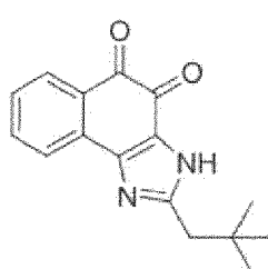
Verbindung 14
