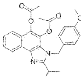
Verbindung 180
