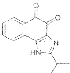
Composé 1
