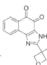
Verbindung 98
