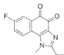
Verbindung 41
