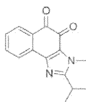
Composé 34
