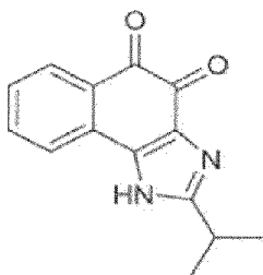
Verbindung 1
