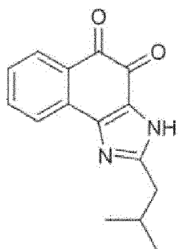
Verbindung 8
