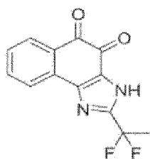
Verbindung 81
