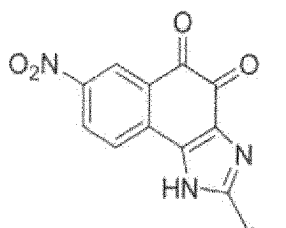
Verbindung 24
