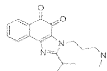
Composé 55
