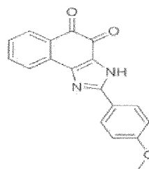
Composé 11
