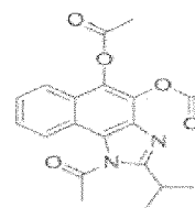
Composé 178
