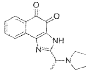
Verbindung 64
