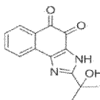
Verbindung 75
