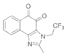
Composé 39
