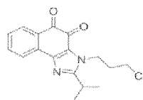
Composé 54
