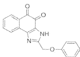
Composé 77
