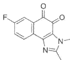
Verbindung 40
