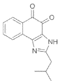
Composé 8
