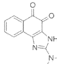
Composé 61
