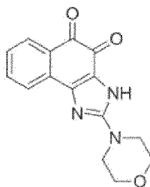
Verbindung 66
