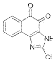
Verbindung 69
