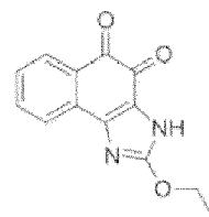
Composé 70
