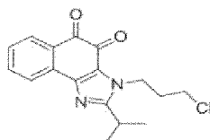
Verbindung 54
