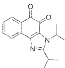
Verbindung 84
