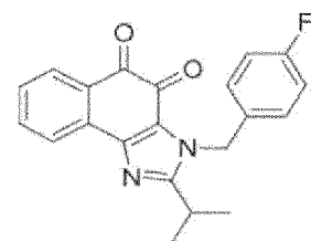
Verbindung 32
