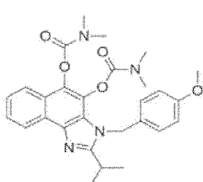
Verbindung 182
