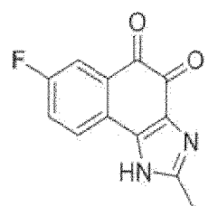
Verbindung 26
