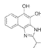
Verbindung 175
