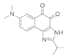
Composé 23
