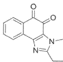
Verbindung 37
