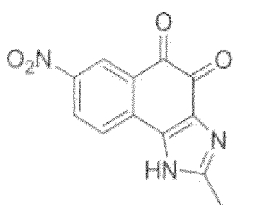
Composé 24
