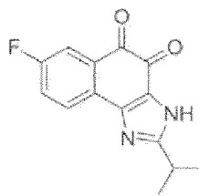
Composé 22
