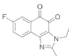
Composé 87
