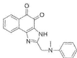
Verbindung 50
