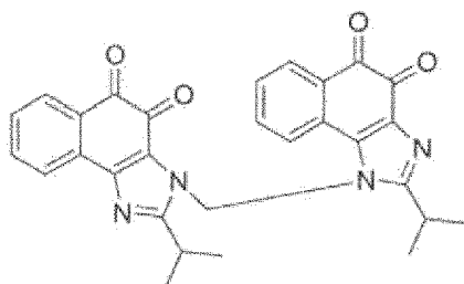
Verbindung 68
