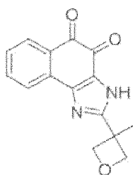
Composé 98
