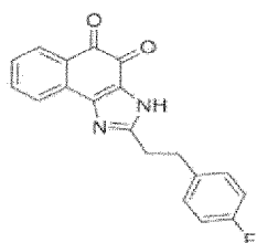
Verbindung 53
