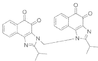
Composé 68
