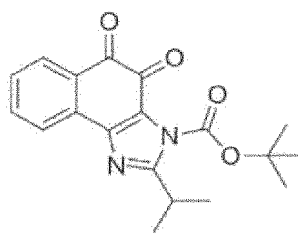
Verbindung 29
