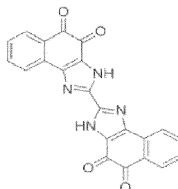
Composé 91
