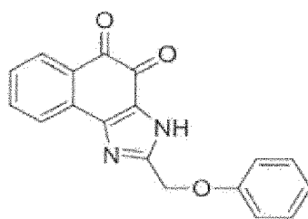
Verbindung 77
