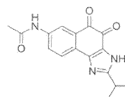
Composé 18
