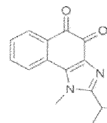
Composé 3
