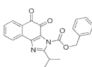
Verbindung 31
