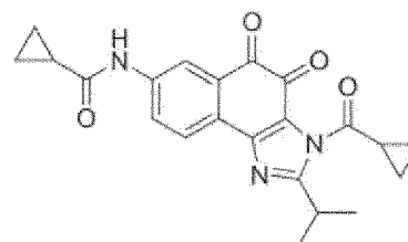
Verbindung 20
