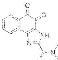
Composé 59
