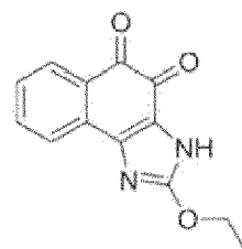
Verbindung 70
