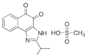
Verbindung 96
