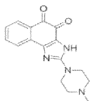
Composé 74
