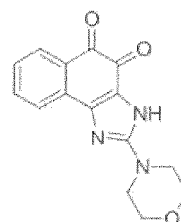
Composé 66
