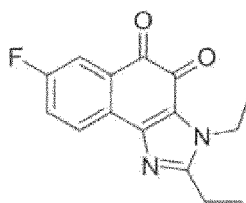
Verbindung 87
