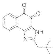
Composé 14
