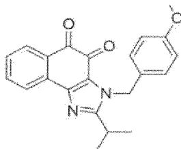
Verbindung 30
