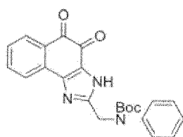
Verbindung 47
