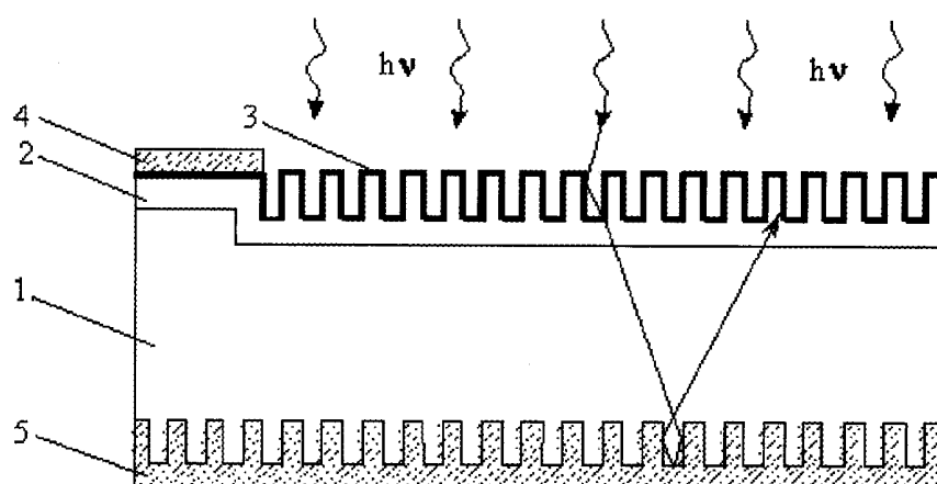
Structura celulei solare
