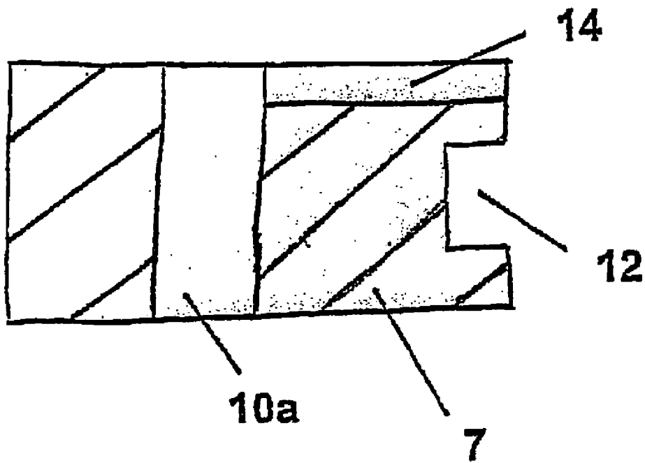
Fig. 1b (Schnitt A-A)
