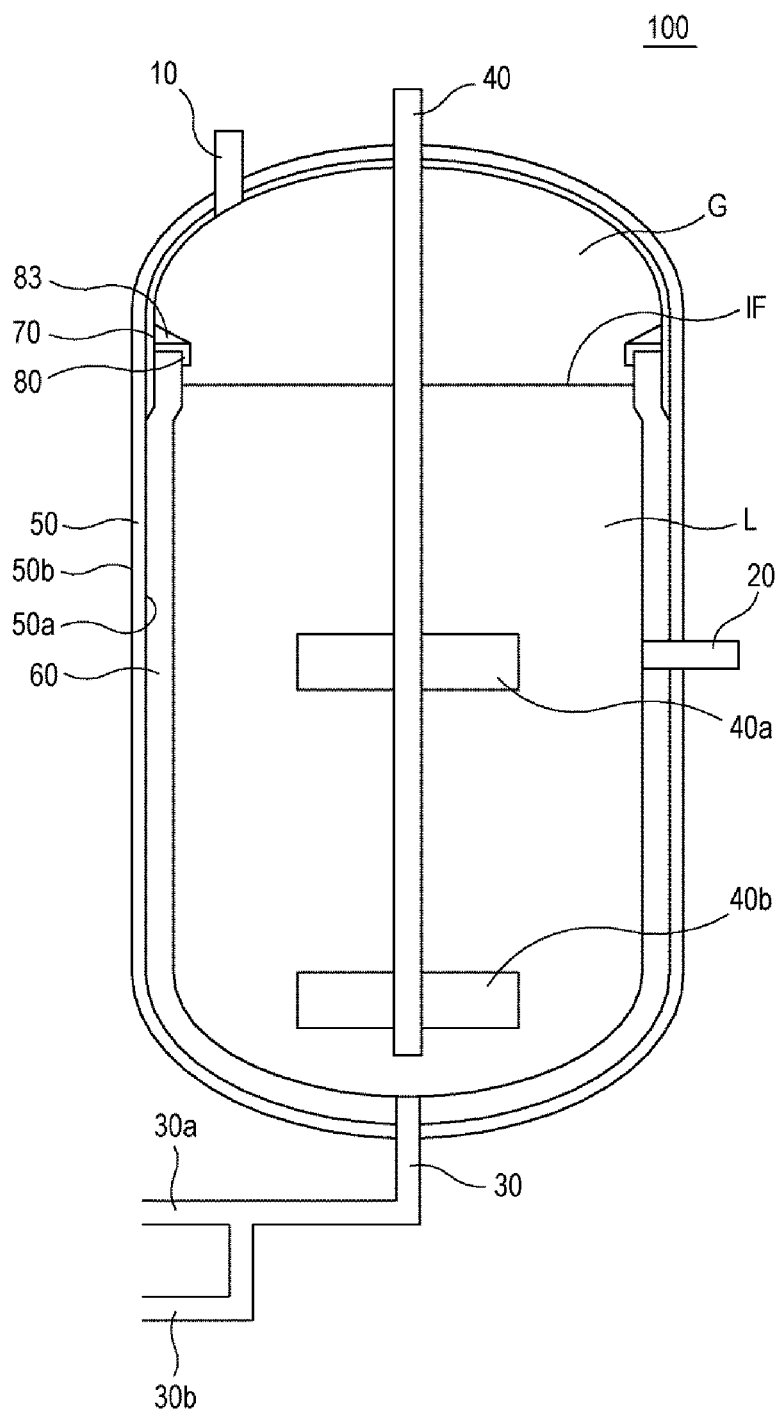
FIG. 4C
