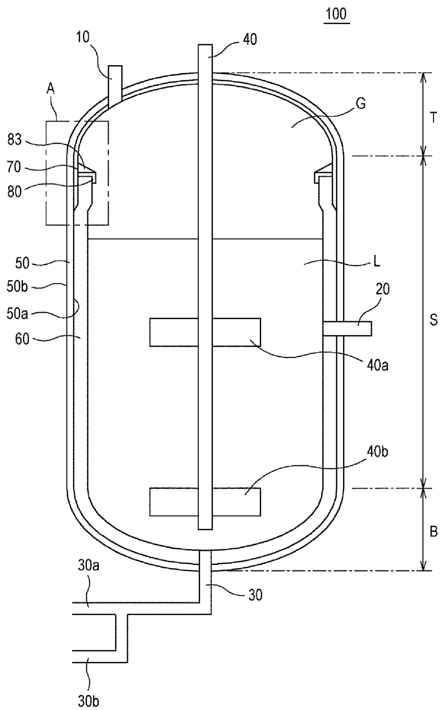
FIG. 1A
