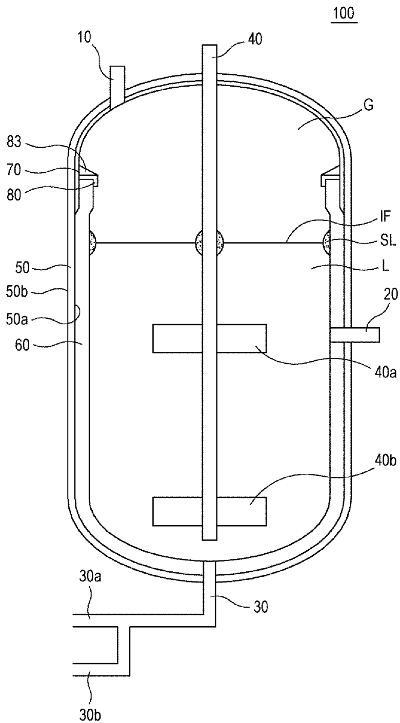
FIG. 4A
