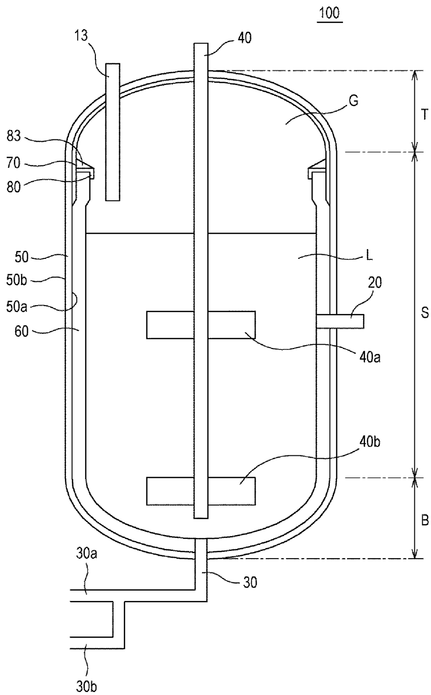
FIG. 1B
