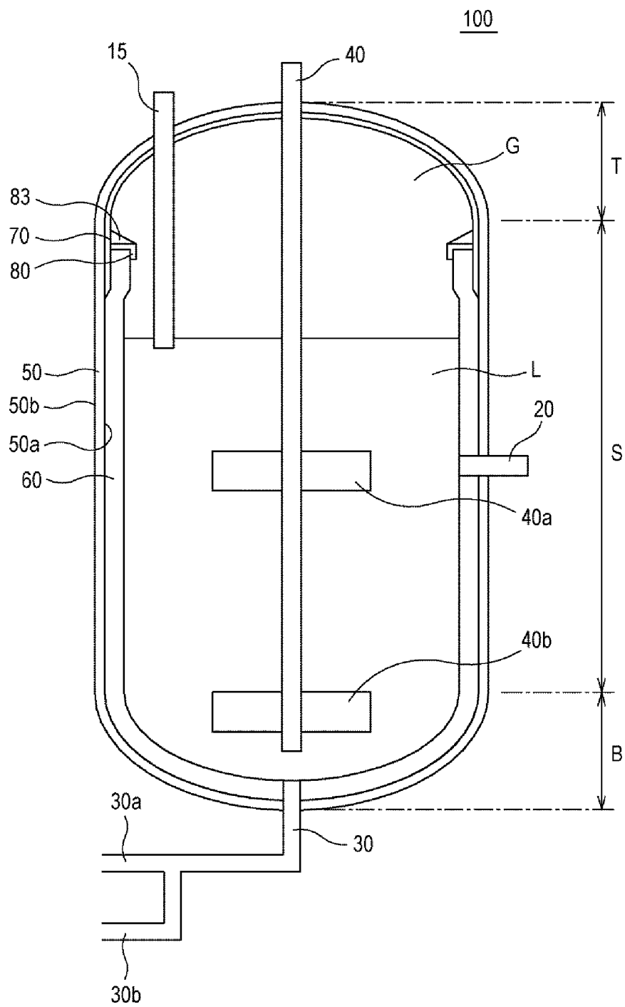
FIG. 1C
