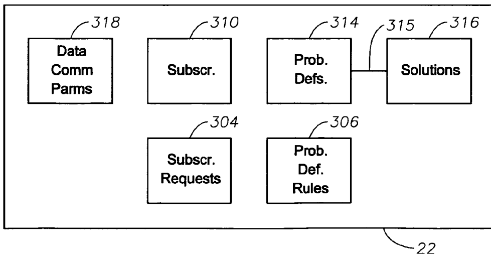
Fig. 2 Database
