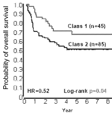
GSE4573 dataset
