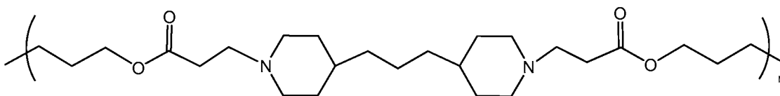
poly 2
