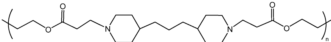
poly 1
