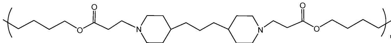
poly 3
