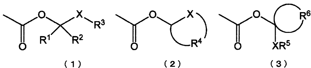
[Chem. 6]
