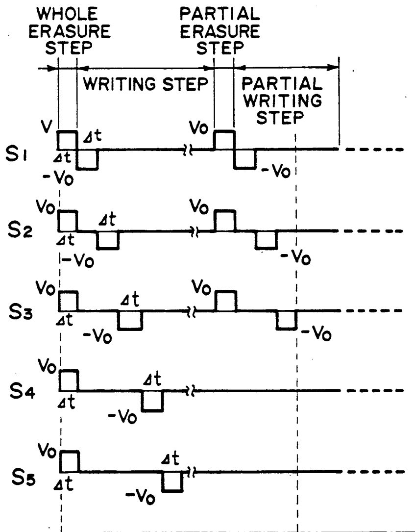
FIG. 13A
