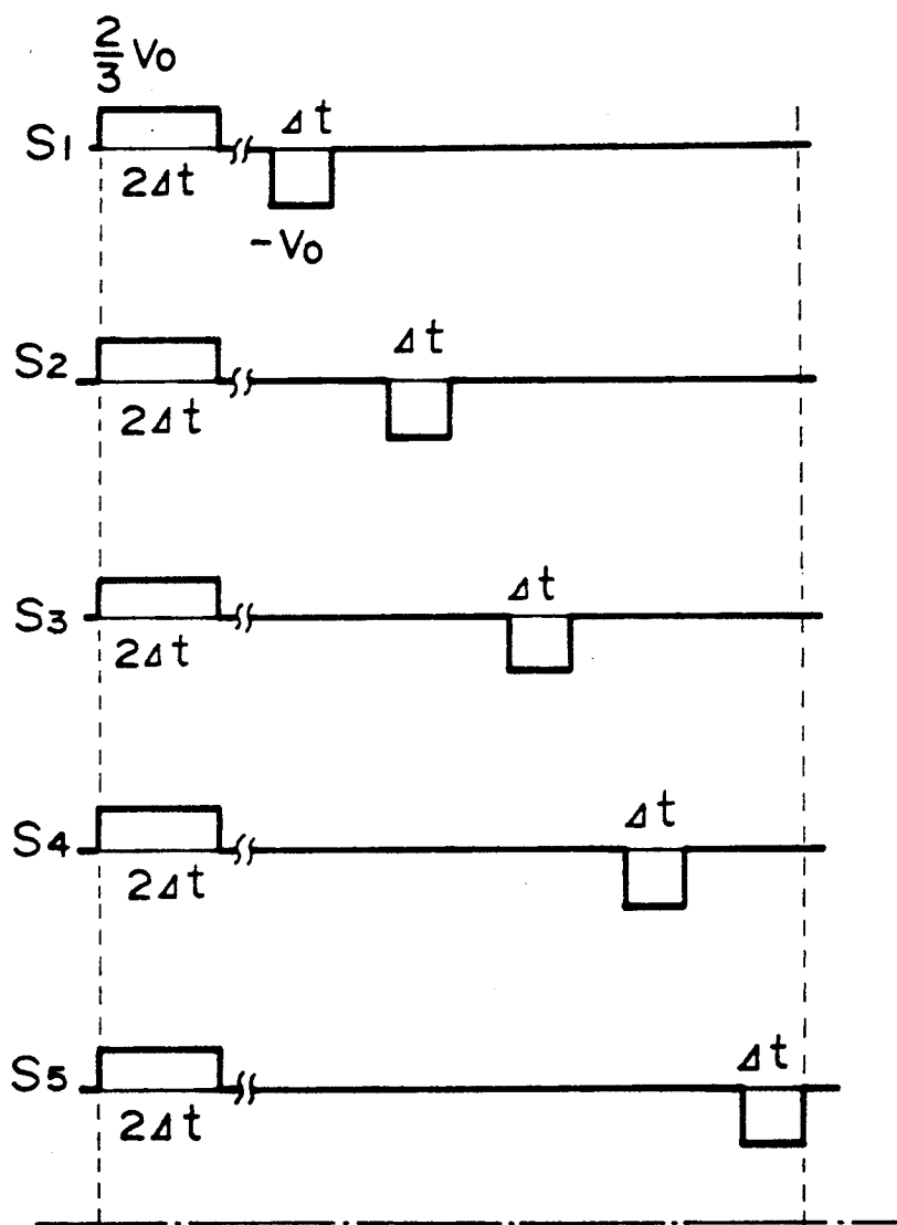
FIG. 10A
