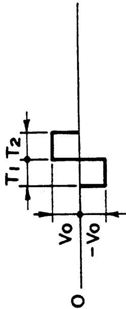
FIG. 5A(d)
