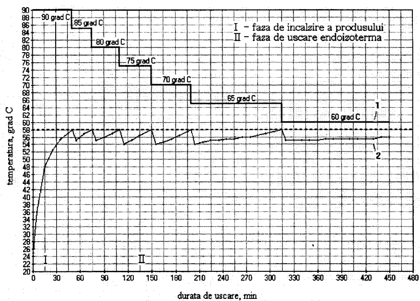
Fig. 1. Diagrama de uscare endoizotermă și termograma tomatelor: 1 – temperatura agentului de uscare, 2 – temperatura produsului
