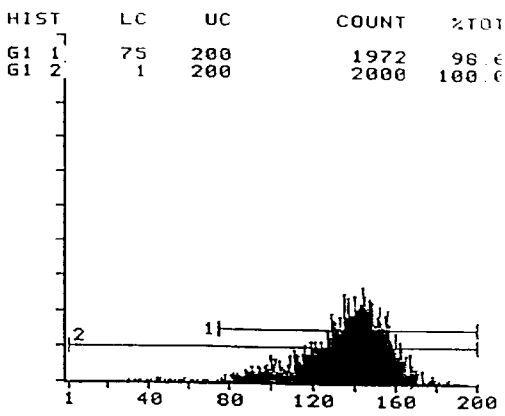
Fig. 19B A431(+MoAb)
