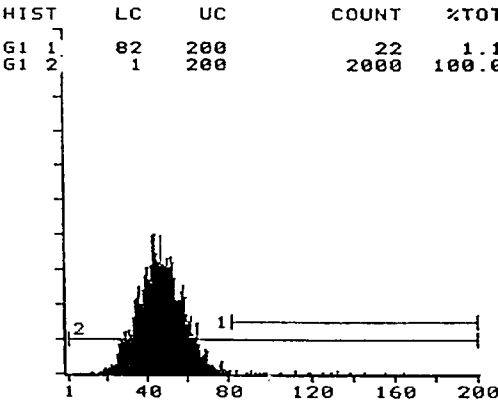
Fig. 19C U-87 MG(-MoAb)
