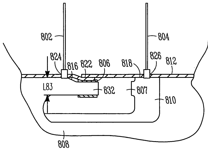
FIG. 8C
