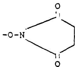
Oxysuccinimide
