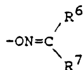
Oxime
