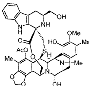
Formule I.
