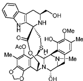
Formel I.
