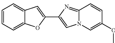
2-(1-benzofuran-2-yl)-6-methoxyimidazo[1,2-a]pyridine
