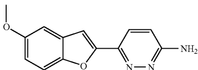
6-(5-methoxy-1-benzofuran-2-yl)pyridazin-3-amine
