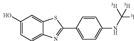
[ 3 H]PIB
