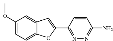
6-(5-methoxy-1-benzofuran-2-yl)pyridazin-3-amine
