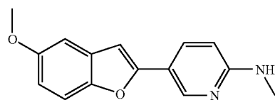
5-(5-methoxy-1-benzofuran-2-yl)-N-methylpyridin-2-amine
