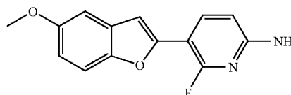
b) 6-Fluoro-5-(5-methoxy-benzofuran-2-yl)-pyridin-2-ylamine
