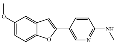
5-(5-methoxy-1-benzofuran-2-yl)-N-methylpyridin-2-amine
