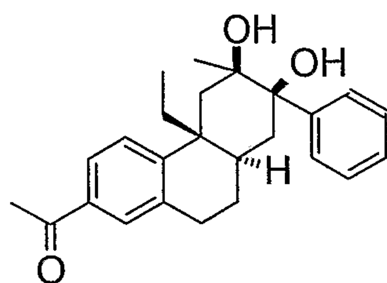
Example 119
