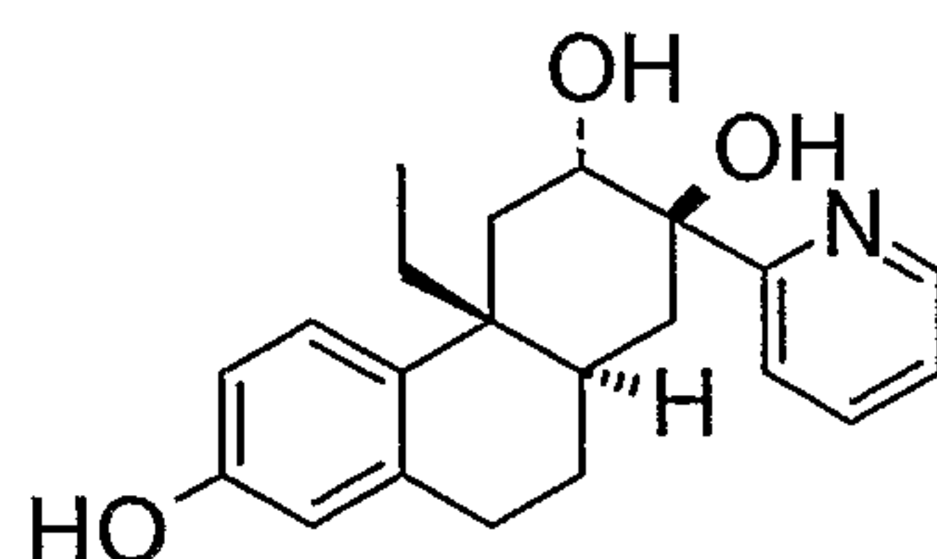
Example 113
