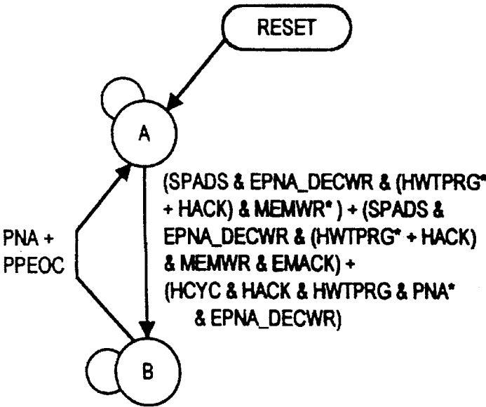
WRPNA STATE MACHINE
