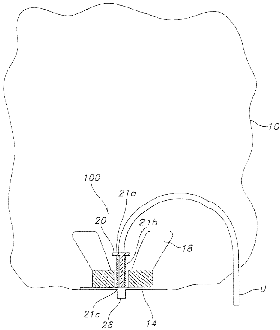
FIG. 10A
