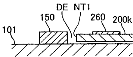
CORTE TRANSVERSAL A-A
