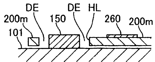
CORTE TRANSVERSAL B-B
