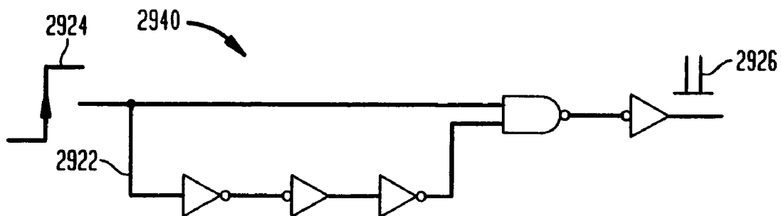
A. RISING EDGE PULSE GENERATOR
