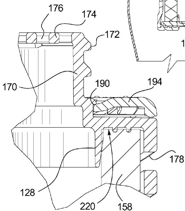
FIG. 20
