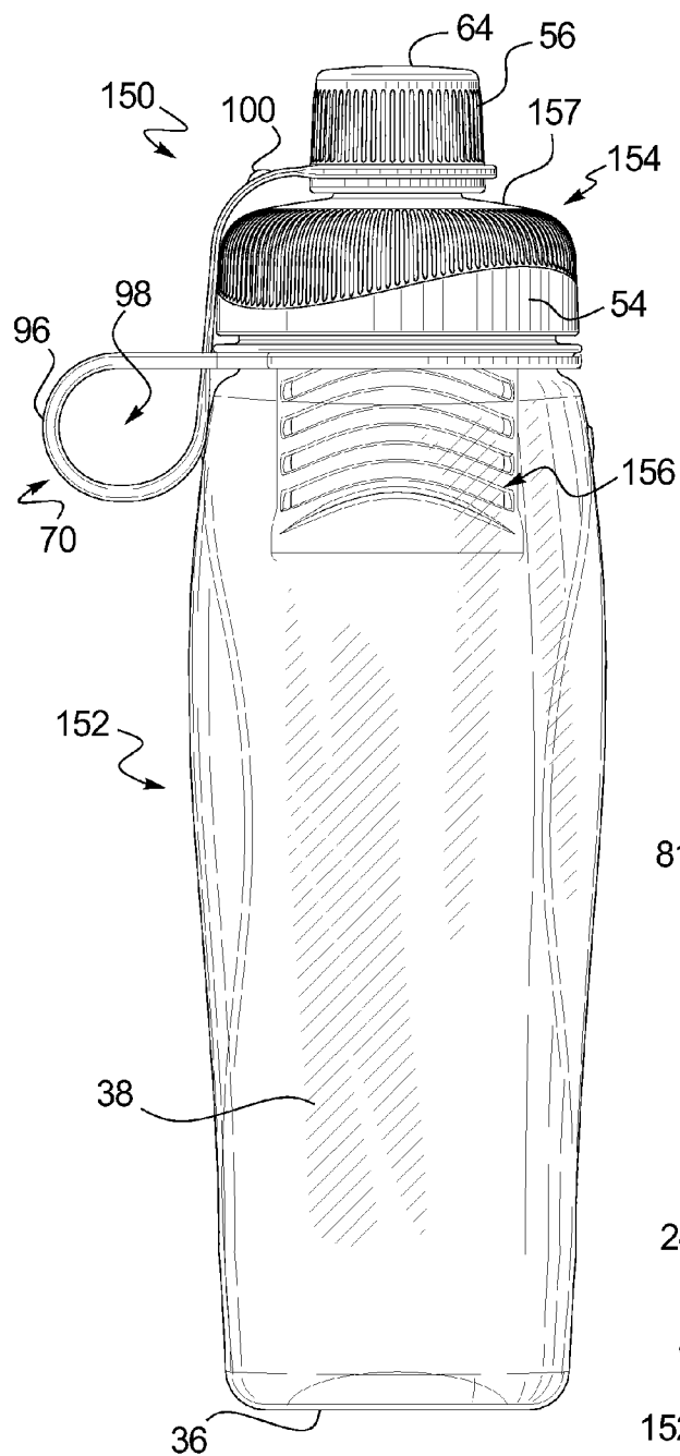
FIG. 14
