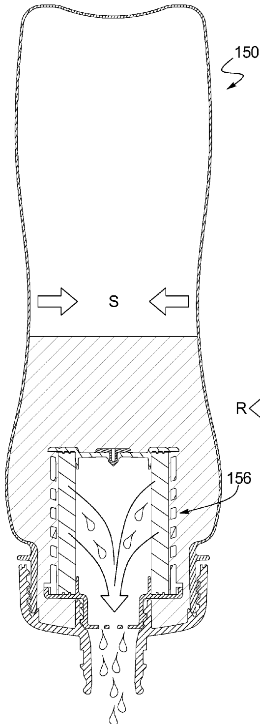
FIG. 27
