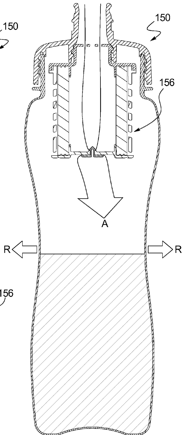
FIG. 28
