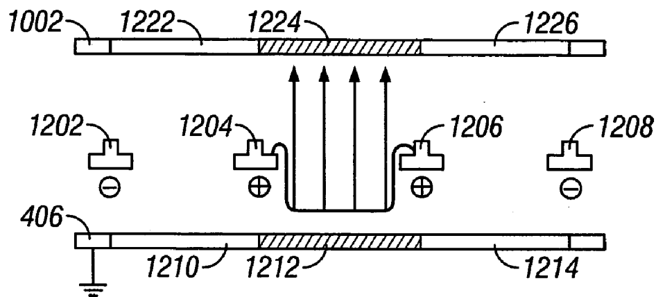
FIG. 12E
