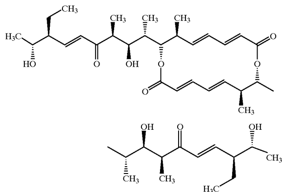
Efomycin M
