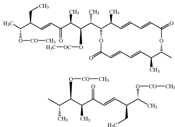
Efomycin T
