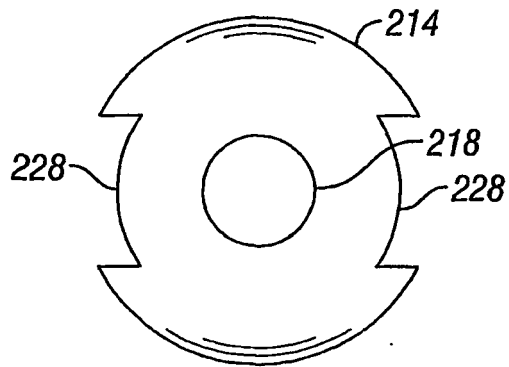
FIG. 18B
