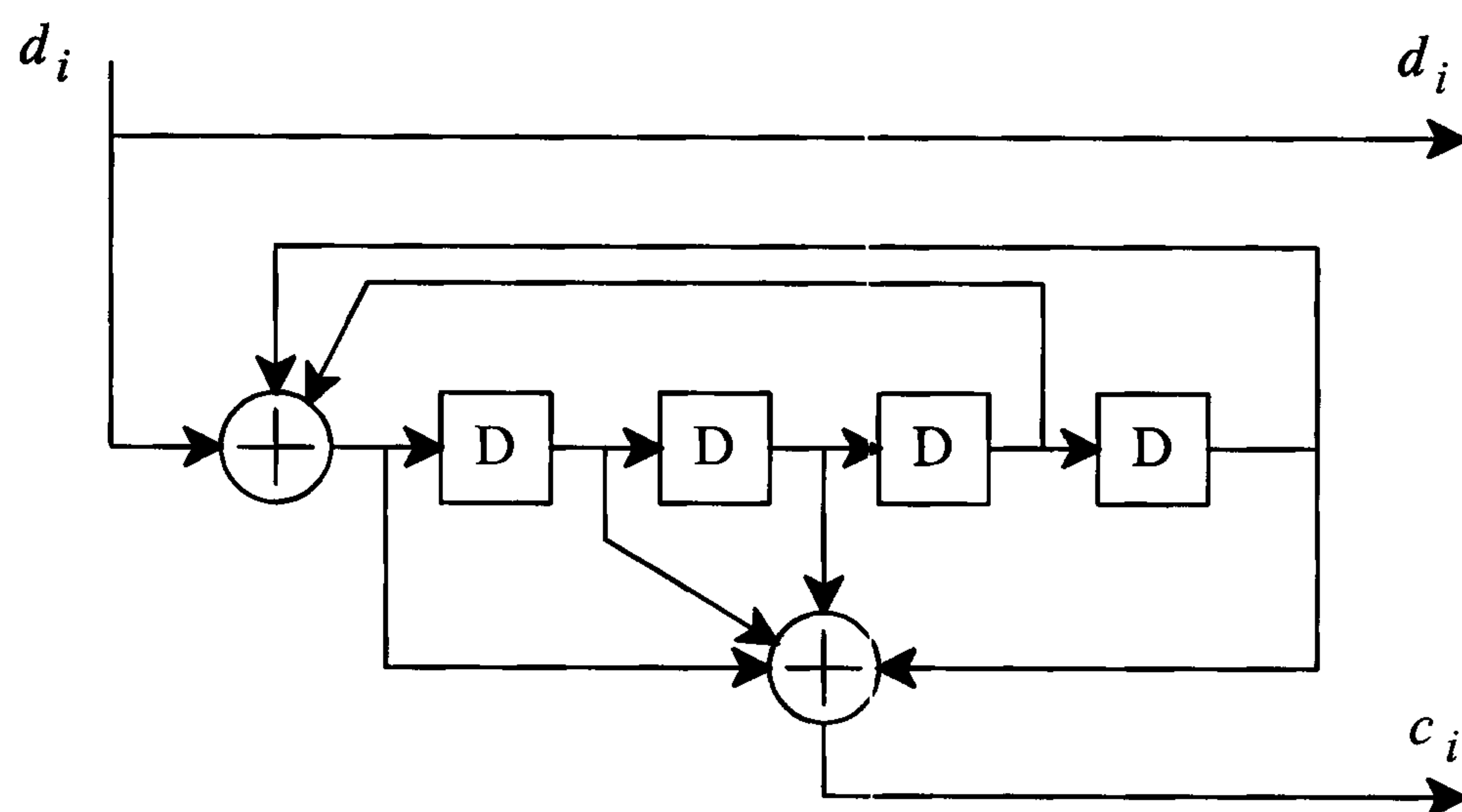
Fig. 2(Prior Art):
