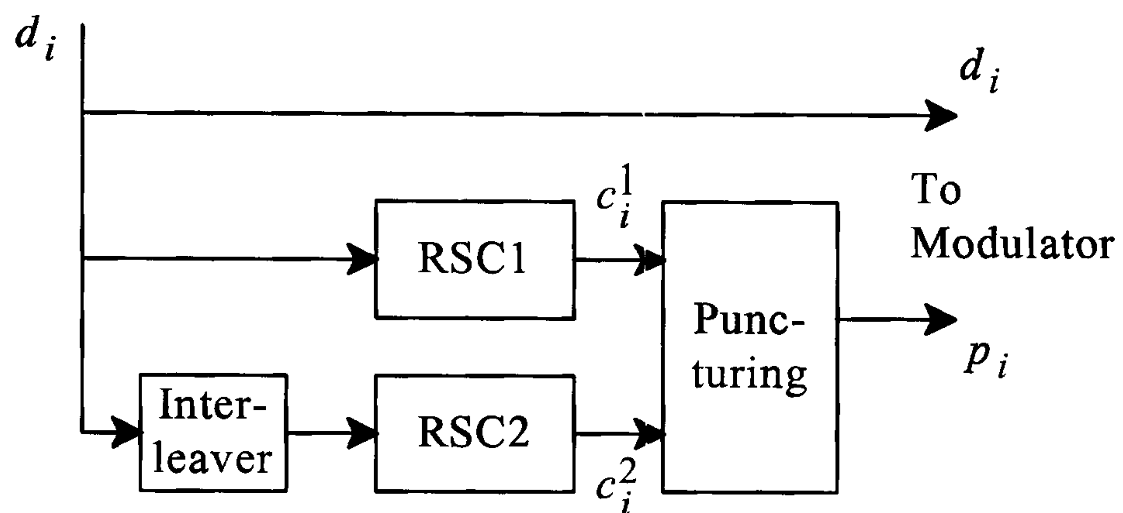
Fig. 1(Prior Art):
