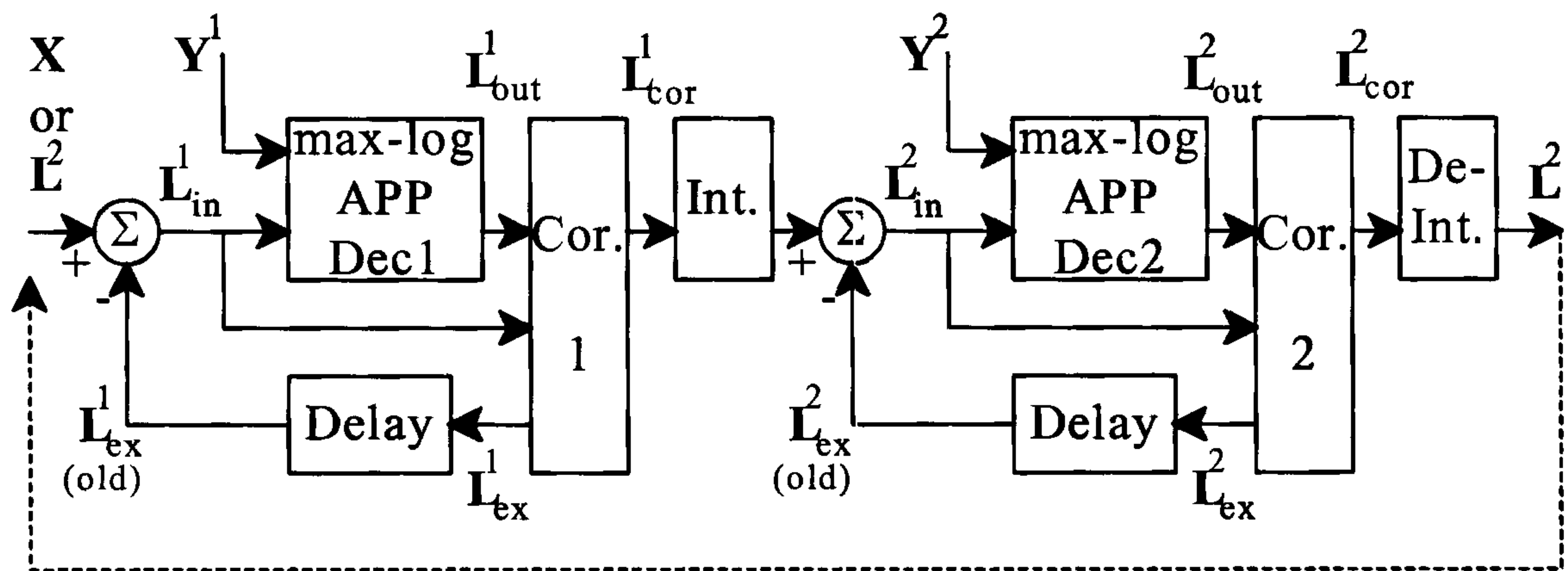
Fig. 4(Prior Art):
