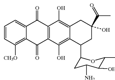
Epirubicin
