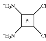
Cisplatin
