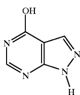
Allopurinol
