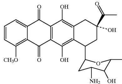
Daunorubicin
