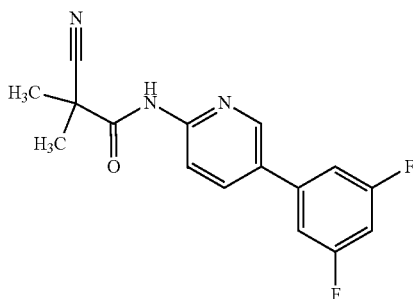
Compound E178
