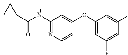
Compound E144
