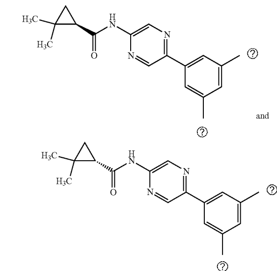
Compounds E231 and E232
