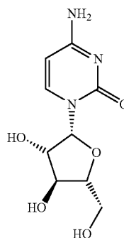
Cytarabine
