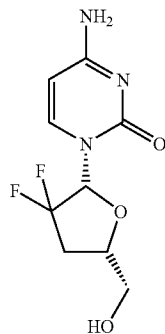
Gencitabine
