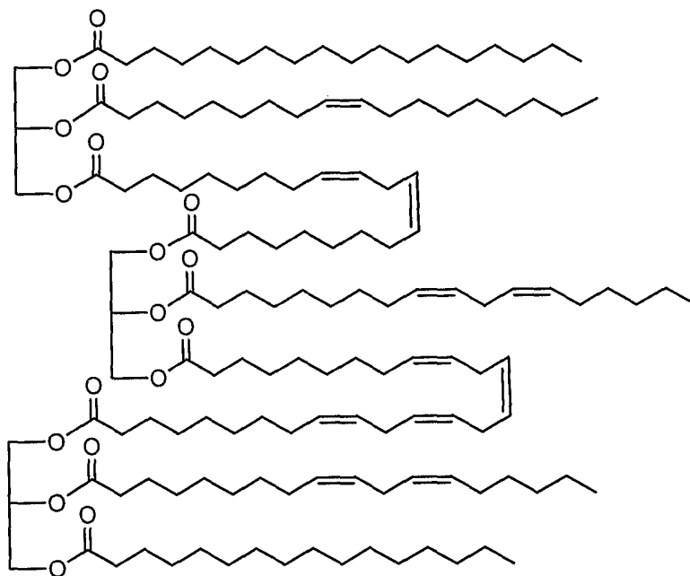
Trimer
