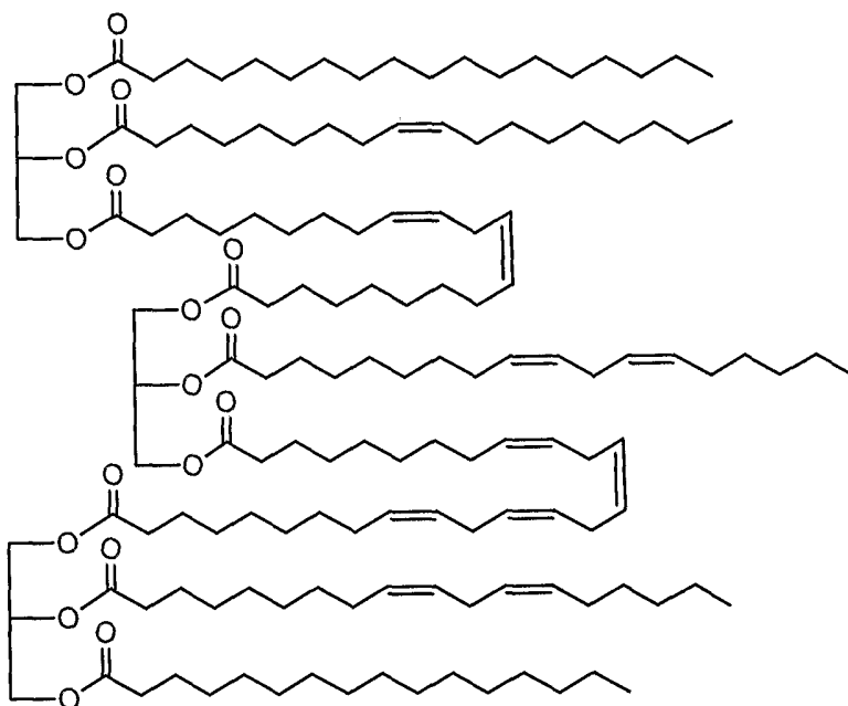
Trimer
