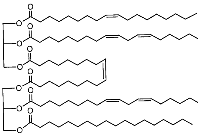
Dimer
