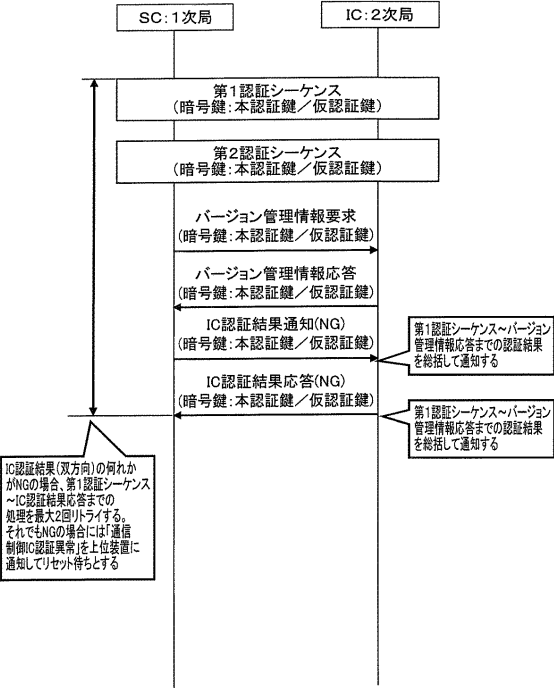
SC-IC間異常系シーケンス 1) 通信制御IC認証異常
