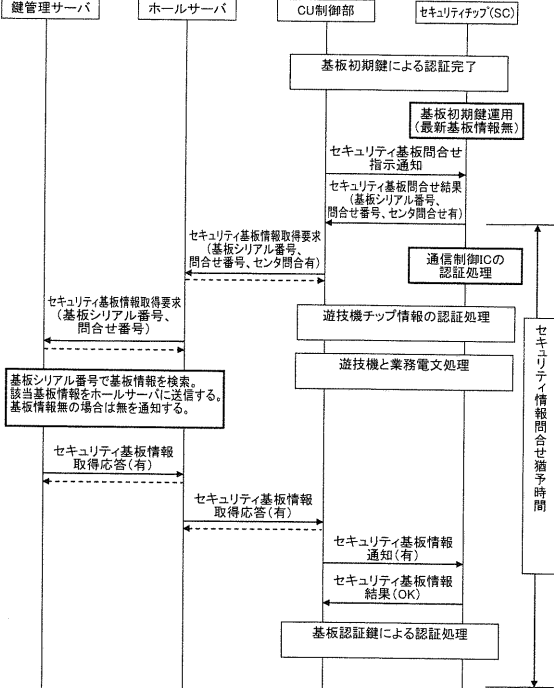
1) 基板初期鍵運用時(ホール設置時)正常取得
