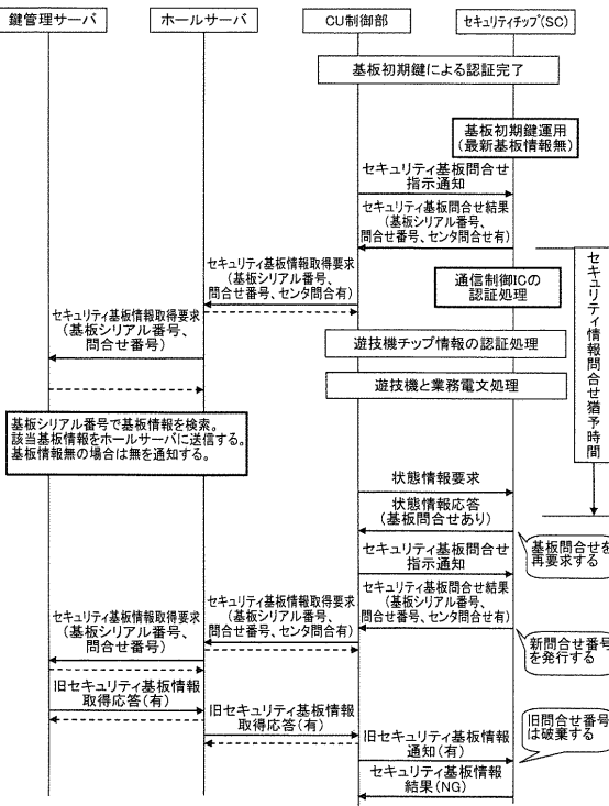
2) 基板初期鍵運用時(ホール設置時)取得タイムアウト
