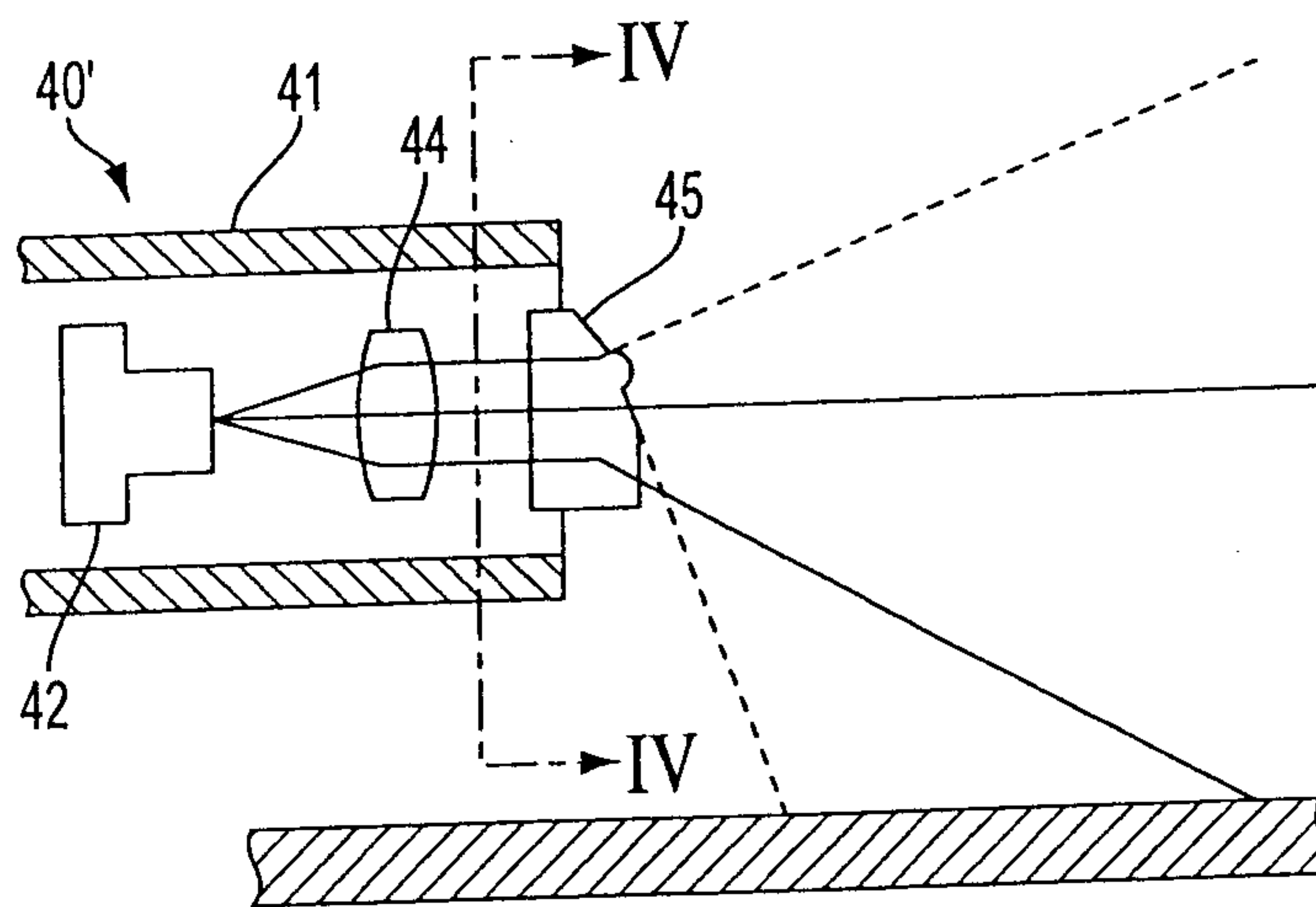
FIG. 4B
