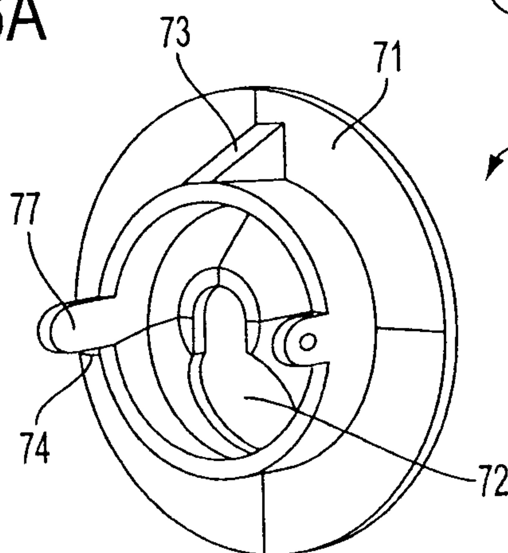
FIG. 7
