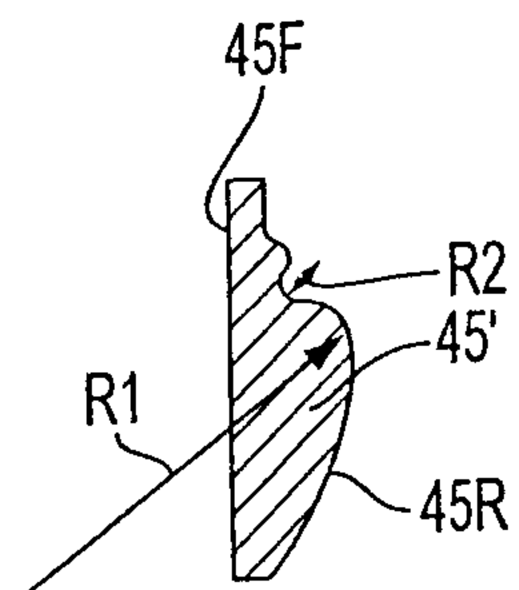
FIG. 4G
