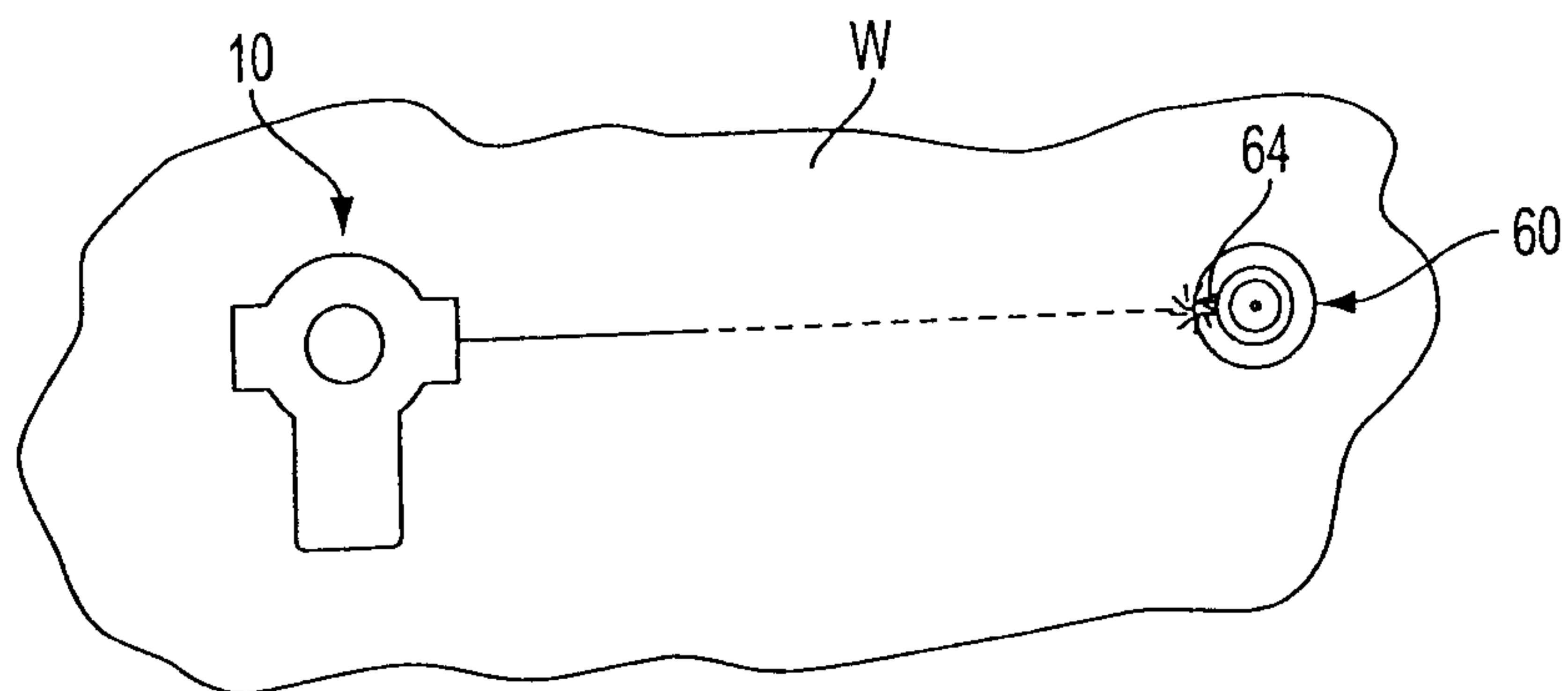
FIG. 5A
