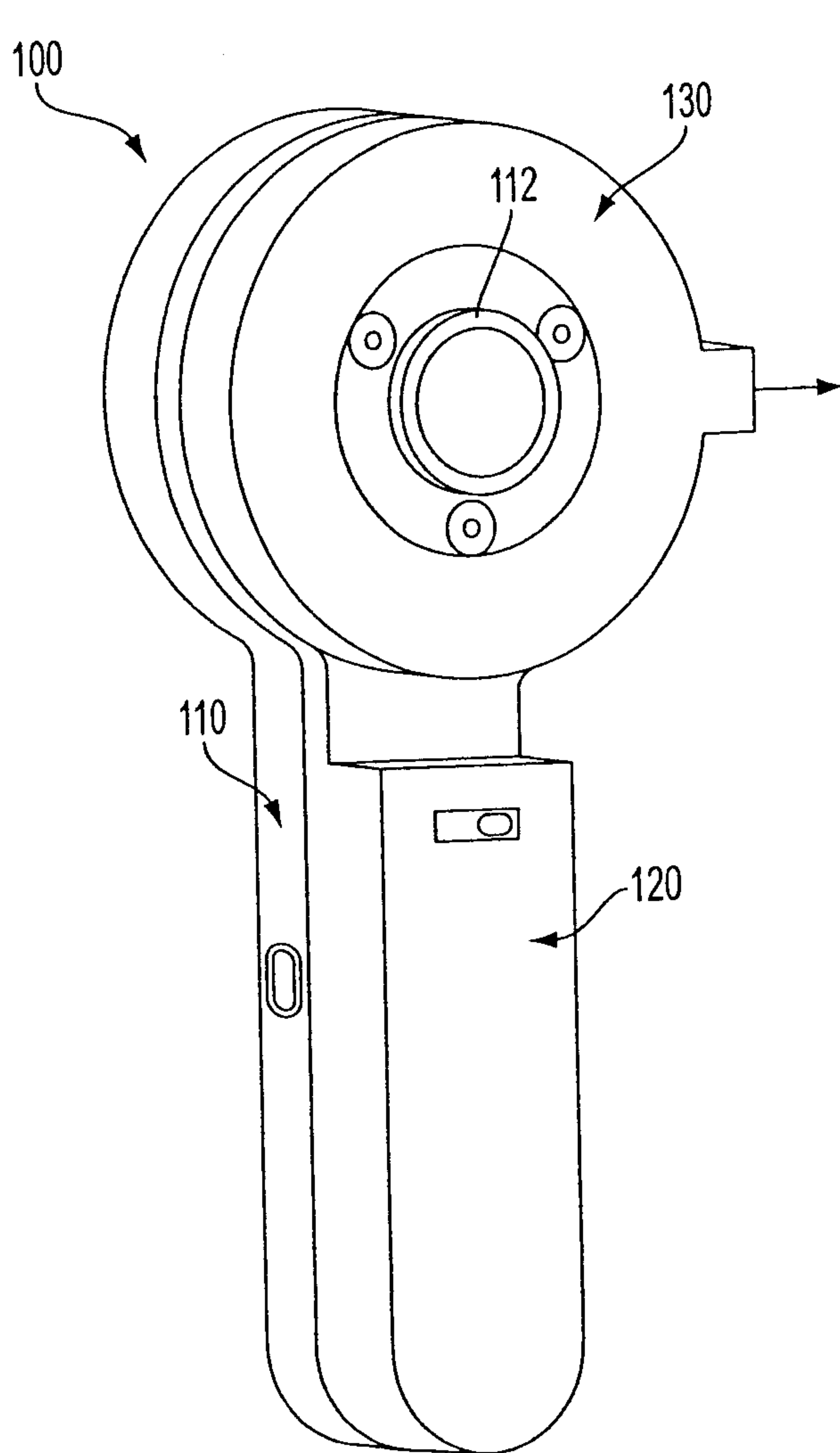
FIG. 10A
