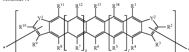
Monomer A
