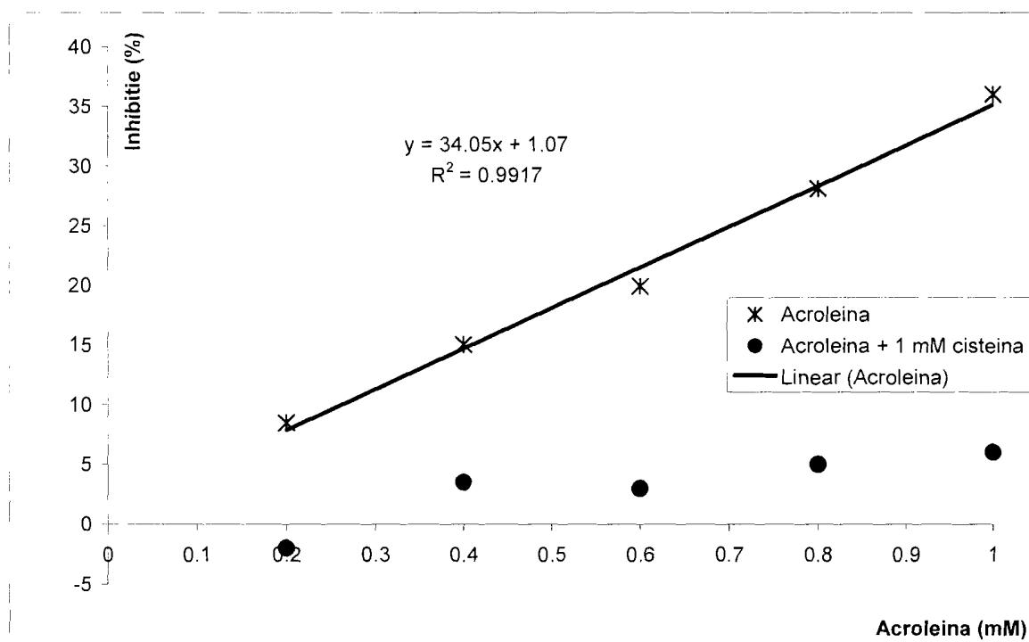
Figura 2. Domeniul liniar al curbei de calibrare folosind soluții standard de acroleină și o comparație cu variația nesemnificativă a activității enzimatică în cazul în care acroleina este amestecată cu cisteina.
