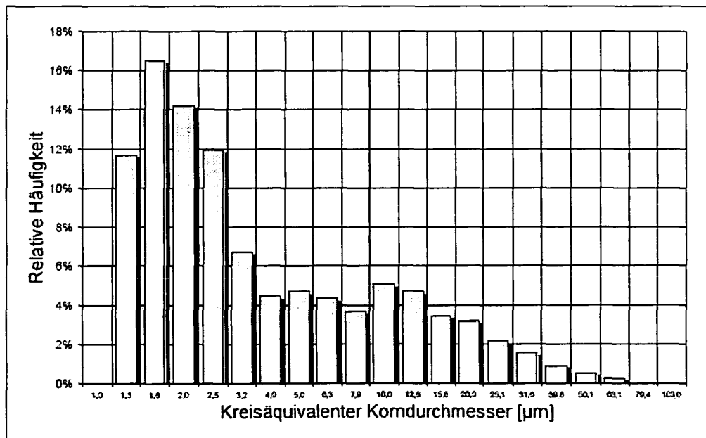
Bild 2: Korngrößenverteilung der Warmwalzvariante "WW2" nach dem 2. Stich
