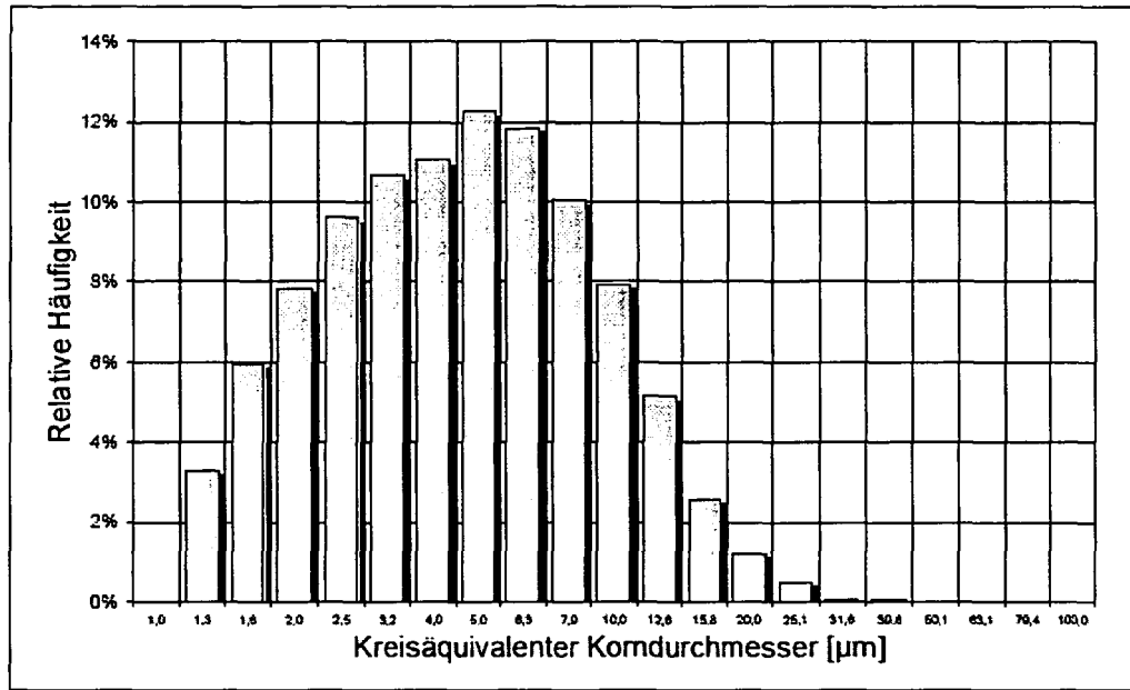
Bild 1: Korngrößenverteilung der Warmwalzvariante "WW1" nach dem 2. Stich
