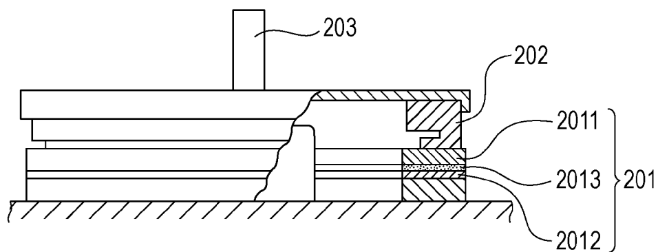
FIG. 6A
