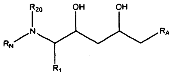
(VI)
