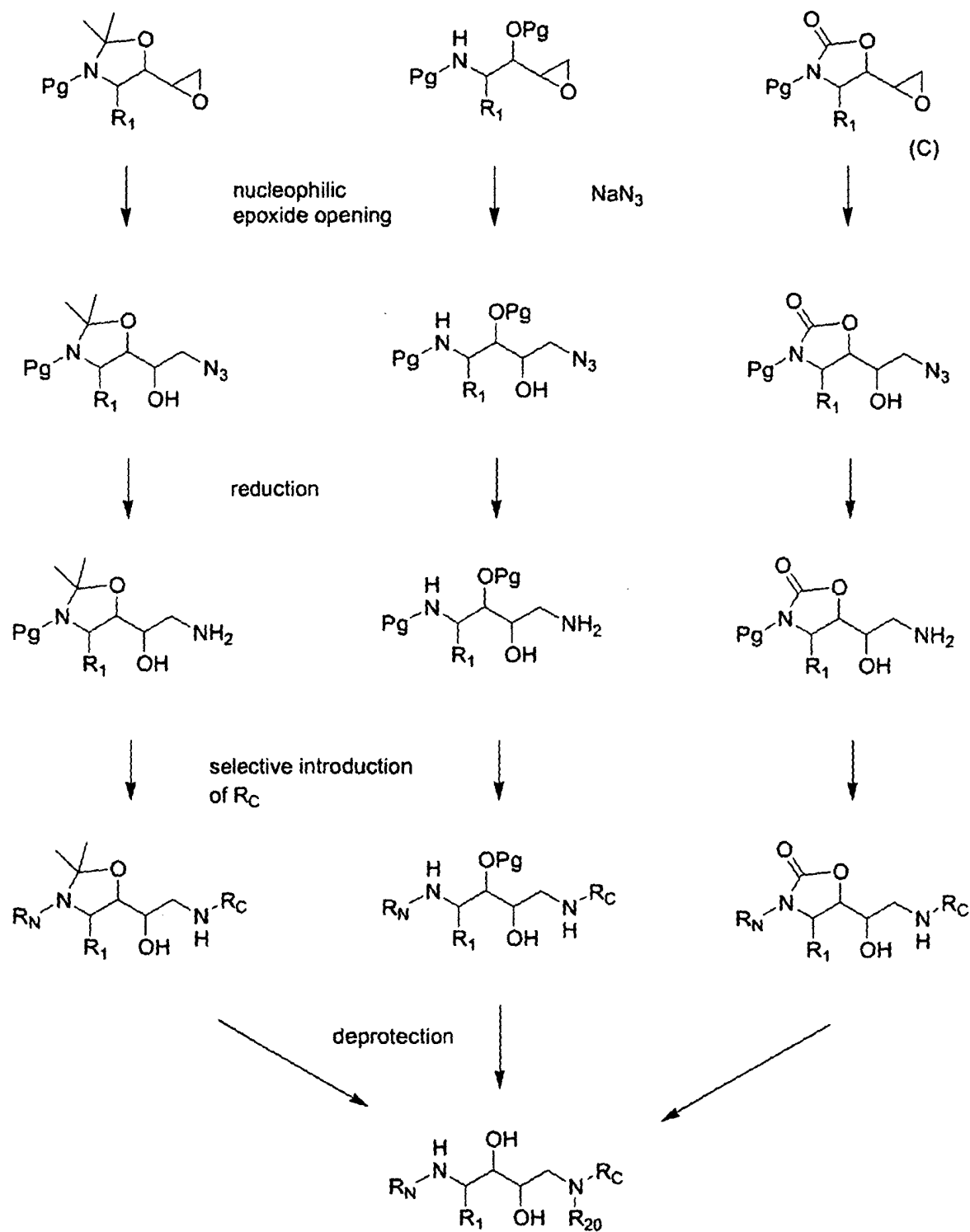
Scheme VI
