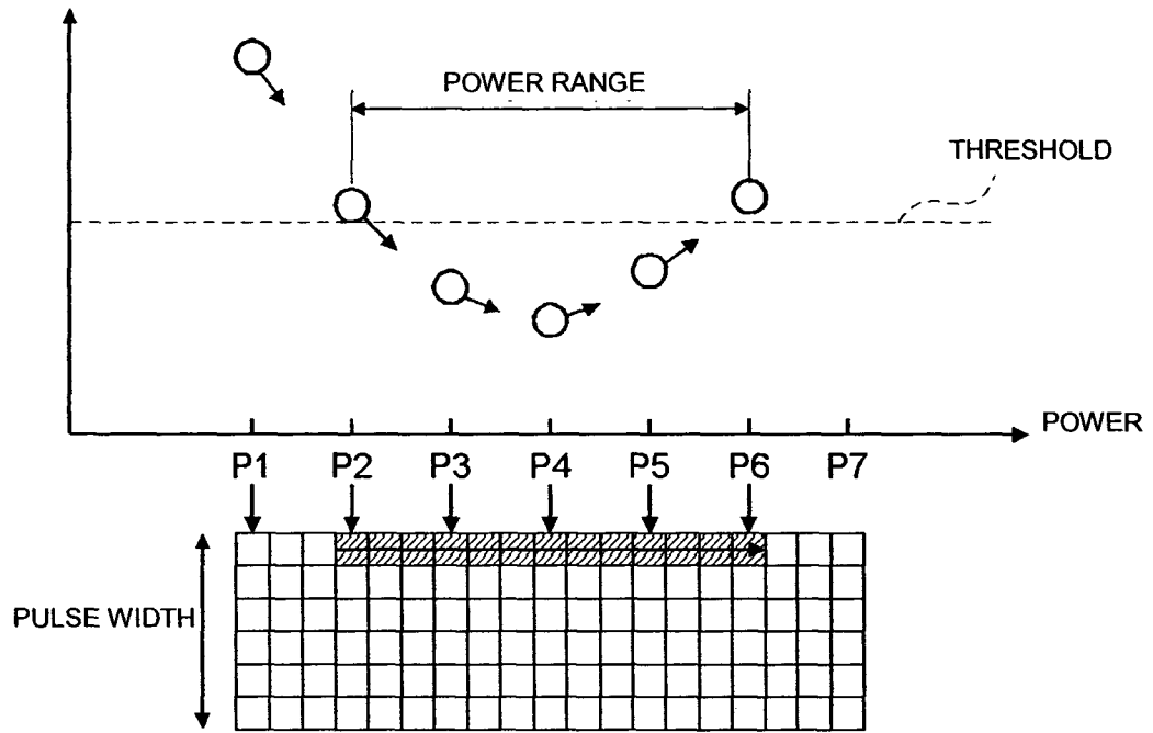
FIG. 17 JITTER
