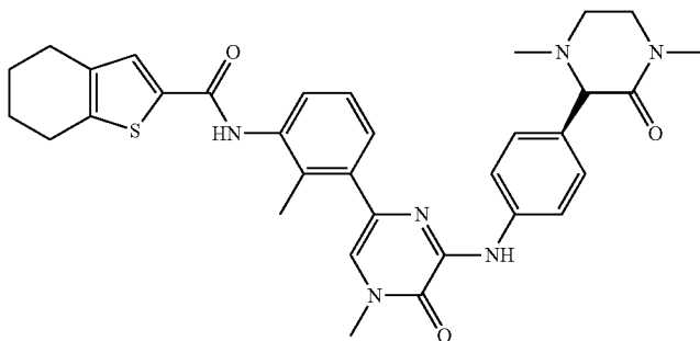
GDC-0834
