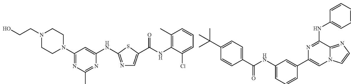
Dasatinib
