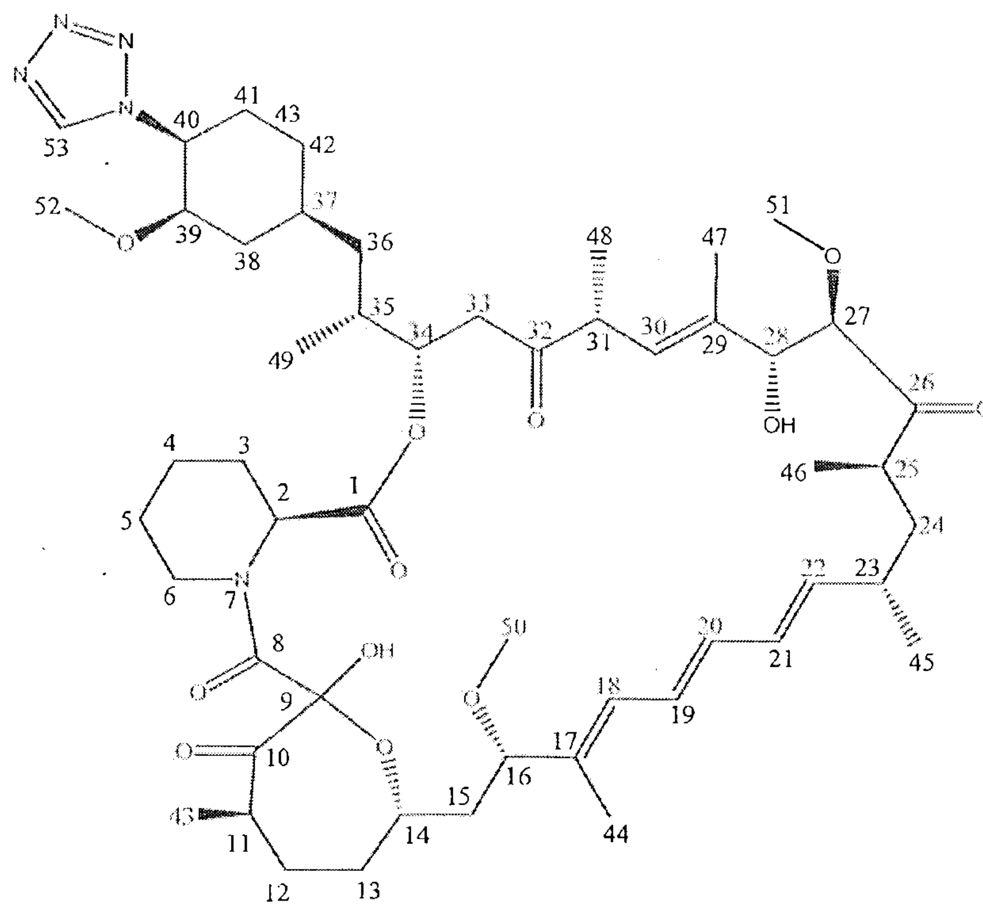
Oxepane 2
