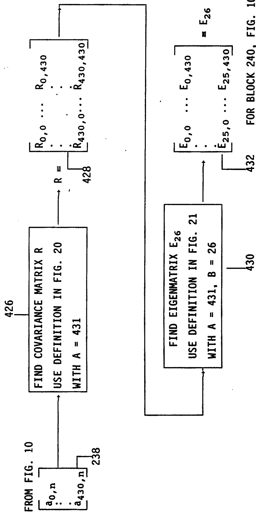
FIG. 22 PARAMETER DEVELOPMENT: EIGENMATRIX E_{26}
