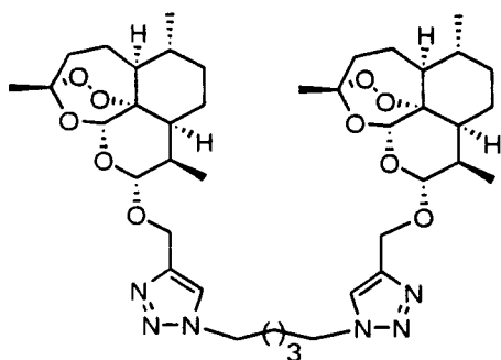
Compound 9a
