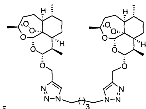
Compound 9a
