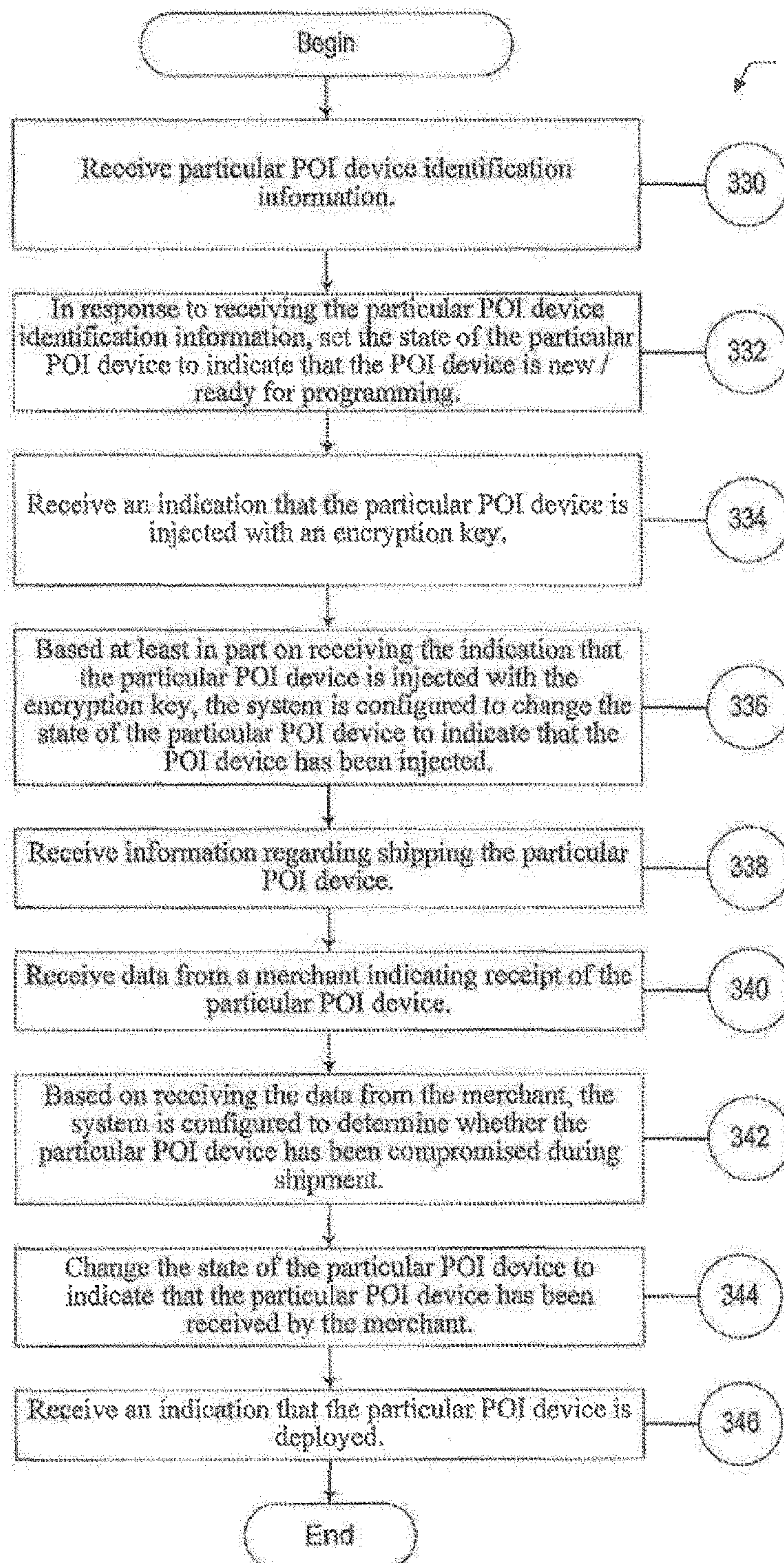
FIG. 3 EXEMPLARY POI HANDLING PROCESS
