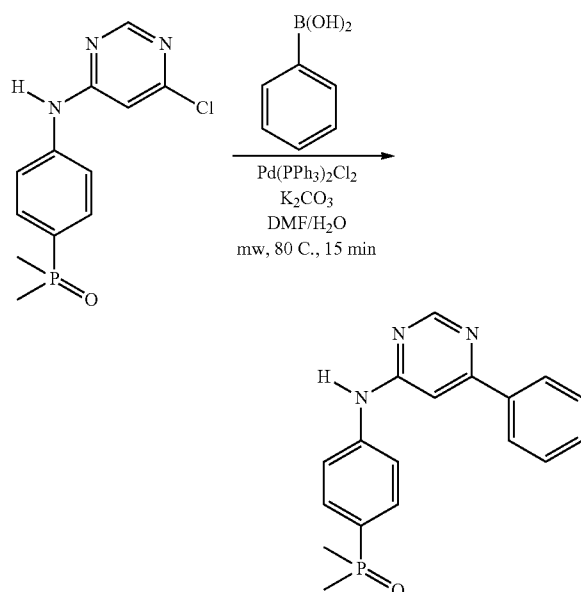
Scheme 31A
