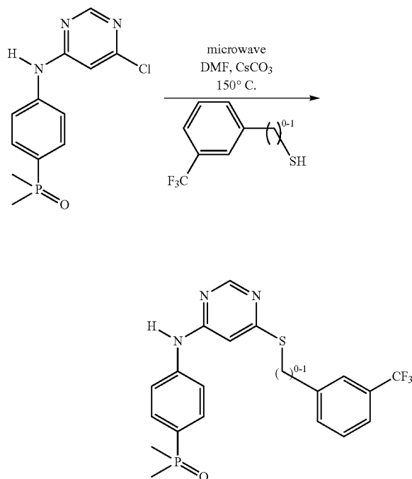
Scheme 30A
