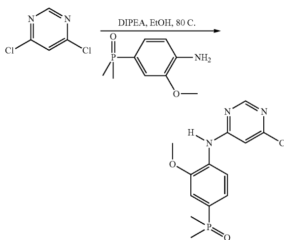
Scheme 25A
